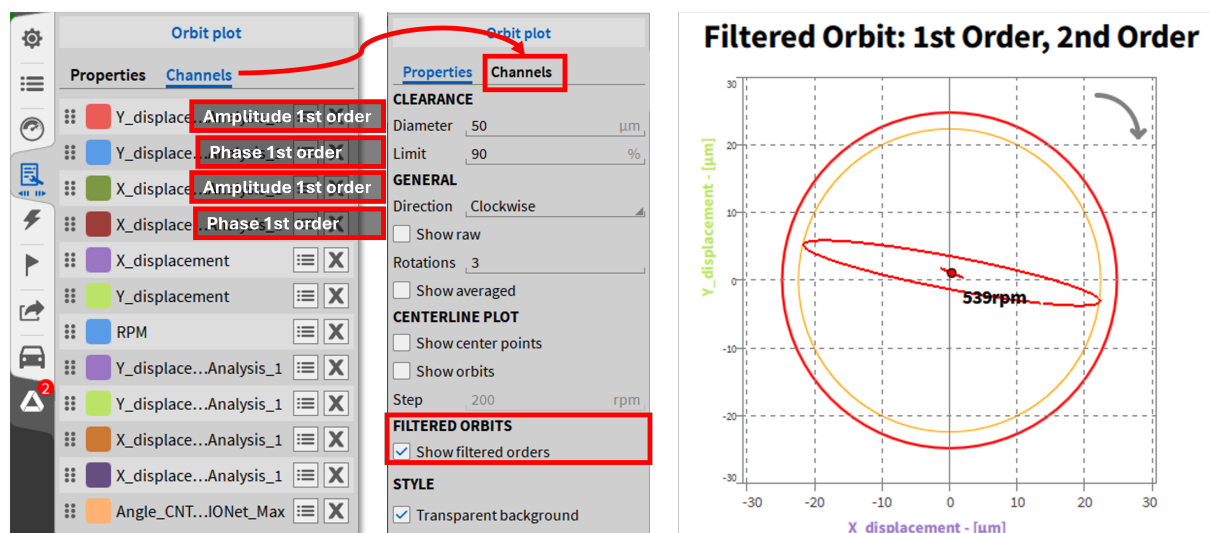
Fig. 8.129: 基于阶次分析的一阶和二阶轨迹实例
