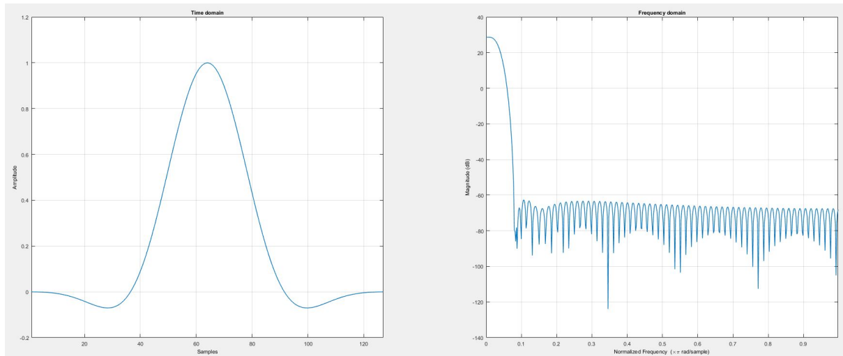
Fig. 8.62: 平顶窗时域和频域特征图 (N = 128)
