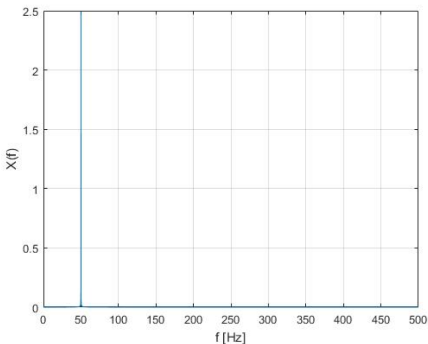
Fig. 8.91: 单侧频谱乘以因数 2
