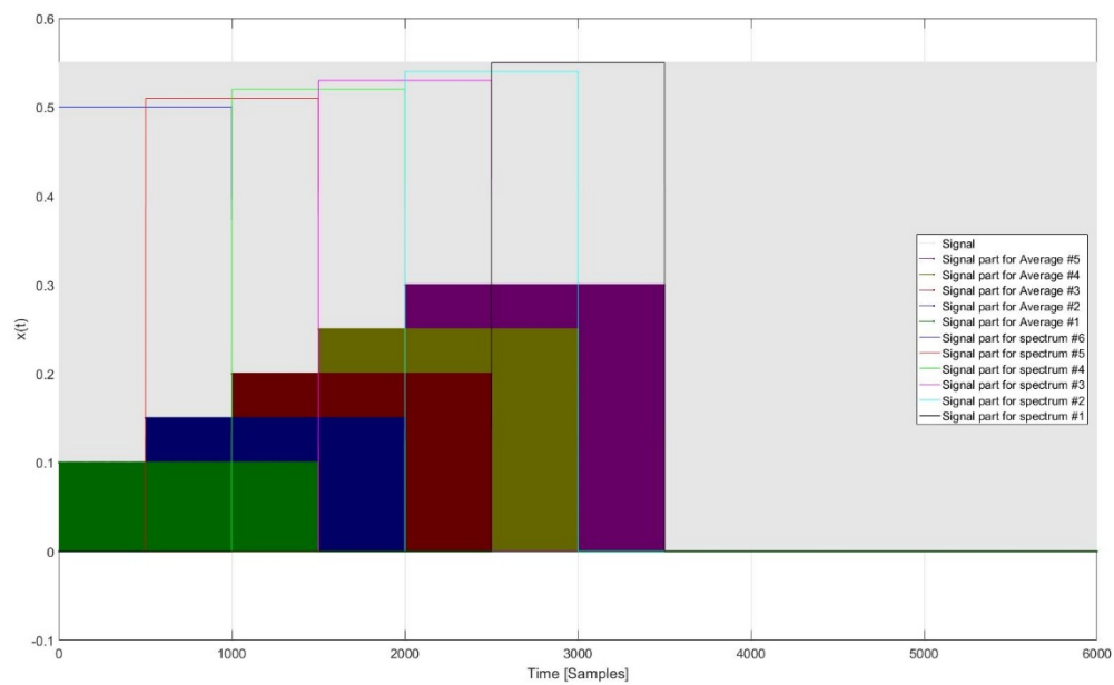
Fig. 8.100: 周期图的时间信号分解, 平均谱为 2, 重叠 50%
