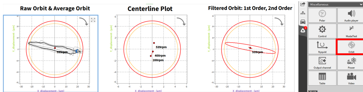
Fig. 8.124: 轴心轨迹图
