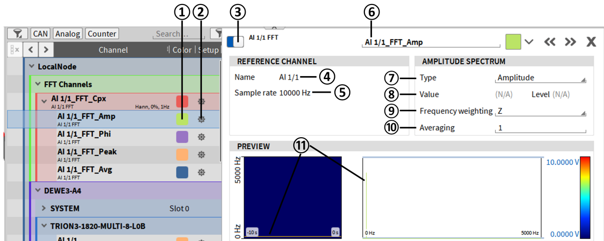
Fig. 7.91: FFT 幅值谱通道设置 - 概览
