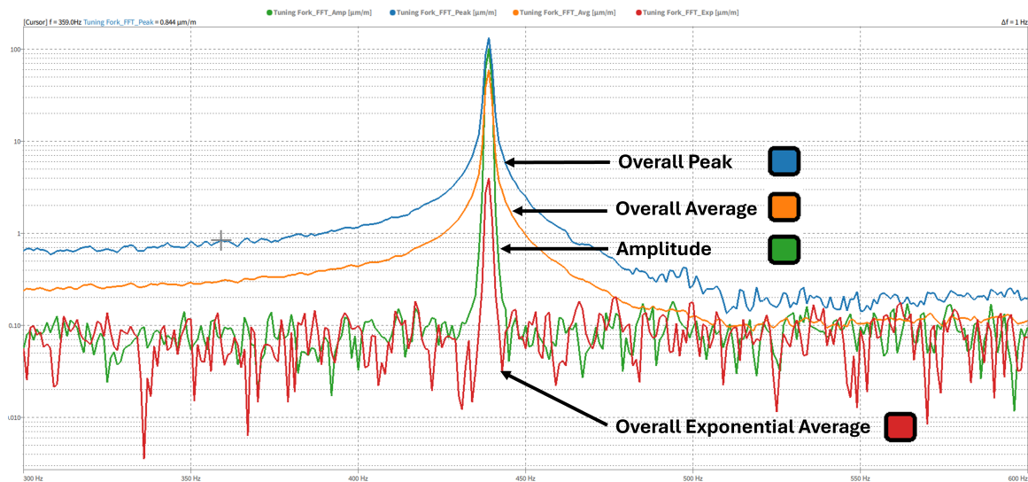
Fig. 7.93: 波谱图中振幅、总体峰值、总体均方根值、总体指数平均值的示例
