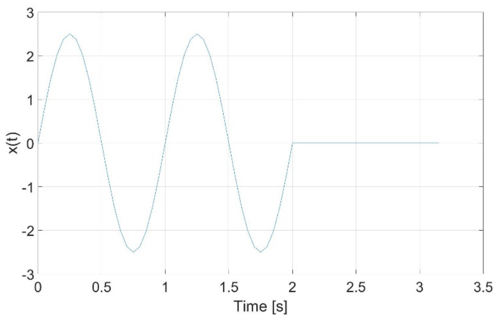
Fig. 8.82: 信号 1 时域图, 零填充至 64 采样点
