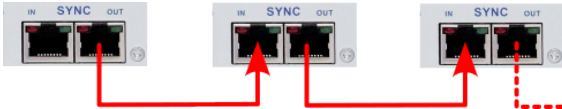
Fig. 15.14: 使用 TRION-SYNC-BUS 同步多个测量单元
