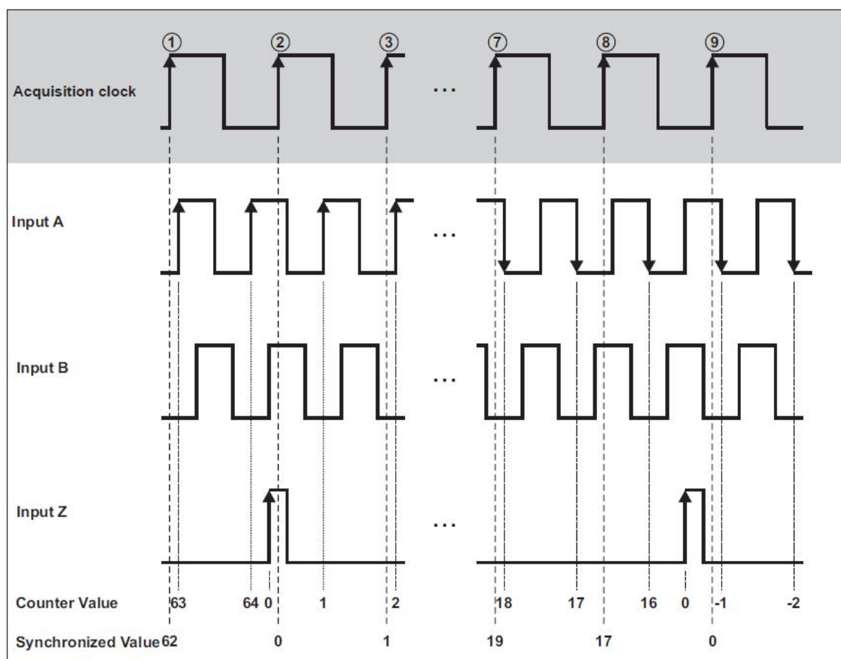
Fig. 7.189: 带有信号 Z 的正交编码器
