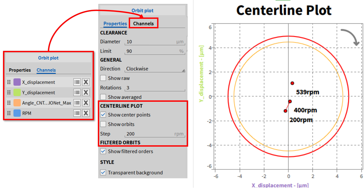
Fig. 8.128: 轴心图示例
