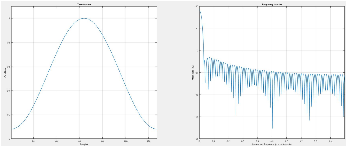
Fig. 8.58: 汉明窗时域和频域特征图 (N=128)
