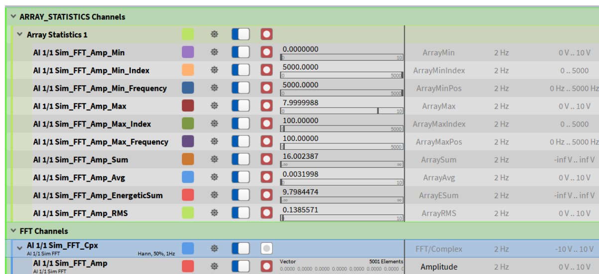
Fig. 7.132: FFT 幅度通道阵列统计示例
