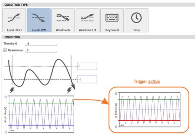
Fig. 9.7: 电平低于阈值触发
