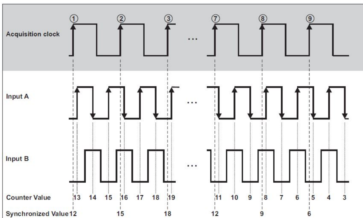
Fig. 7.187: 90 度正交编码器 X2 模式
