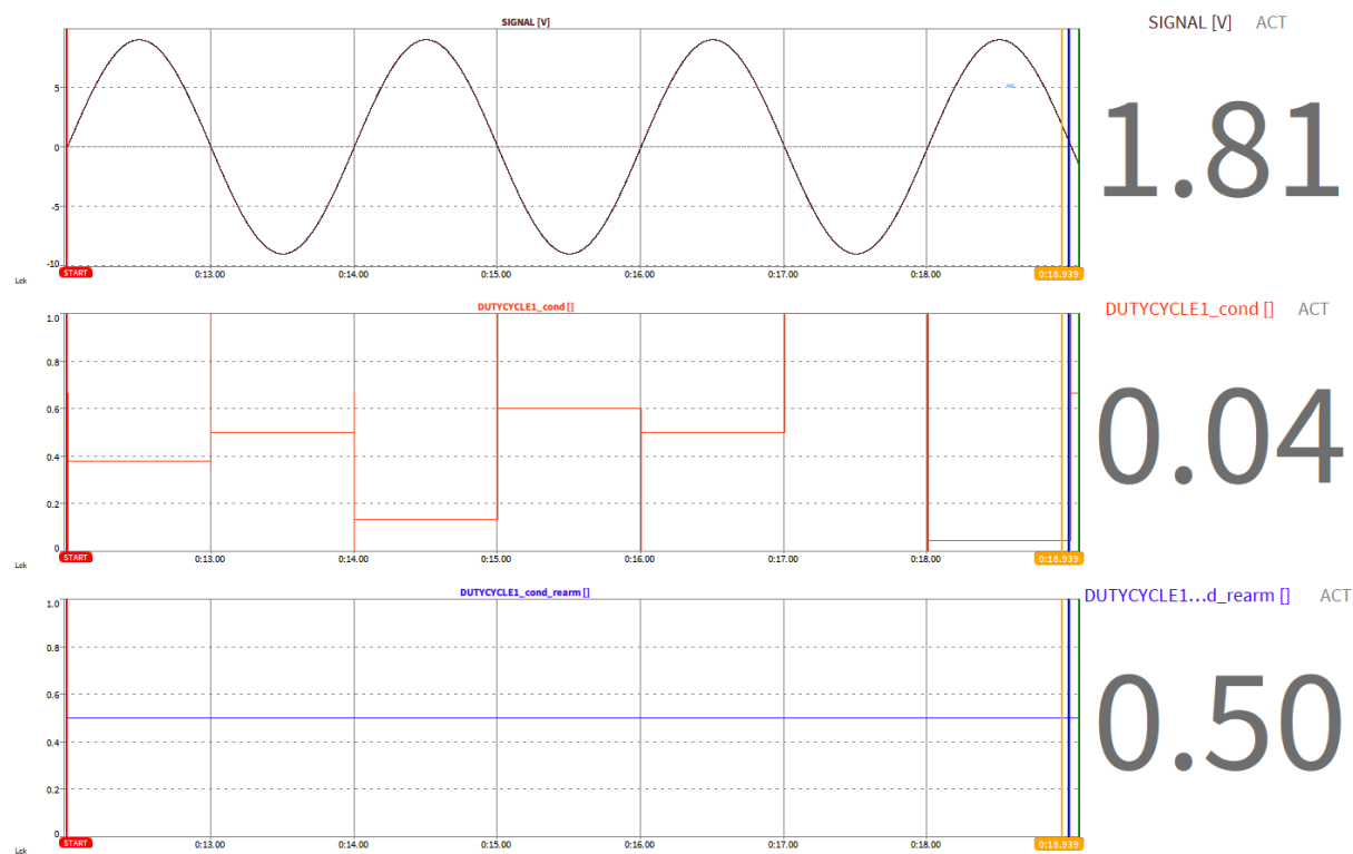
Fig. 7.70: 占空比计算
