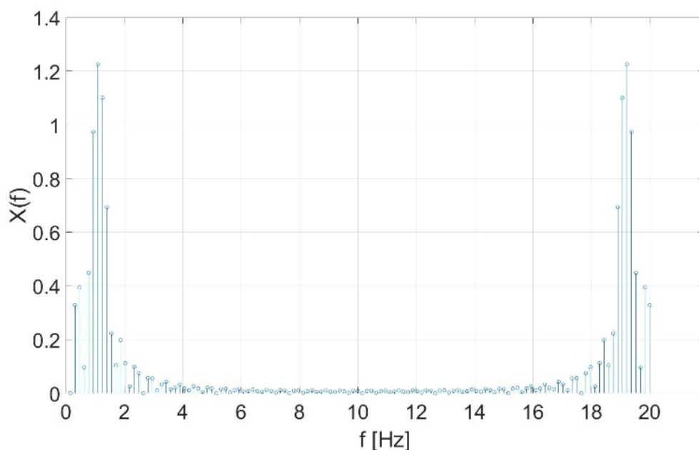
Fig. 8.85: 信号 1 的频谱, 零填充至 128 采样点
