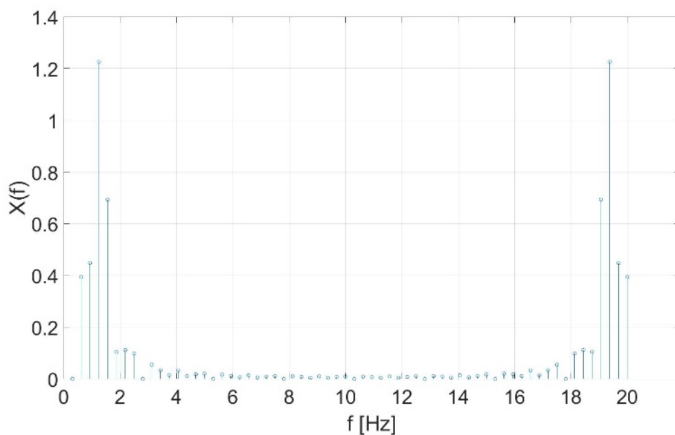
Fig. 8.83: 信号 1 的频谱, 零填充至 64 采样点
