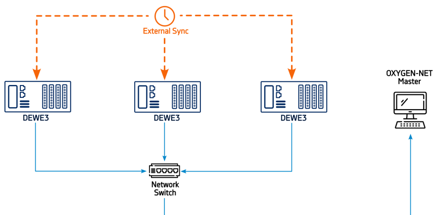
Fig. 15.6: 外部时钟源同步拓扑图
