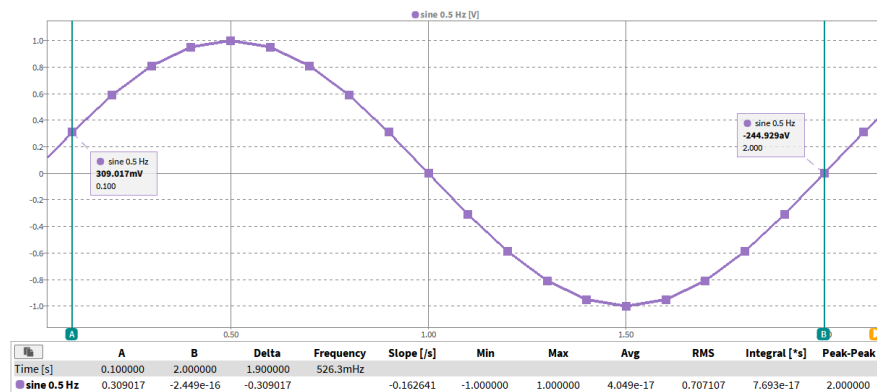
Fig. 8.33: 0.5 Hz 正弦波; 光标 A 在 0.1, 光标 B 在 2.0s
