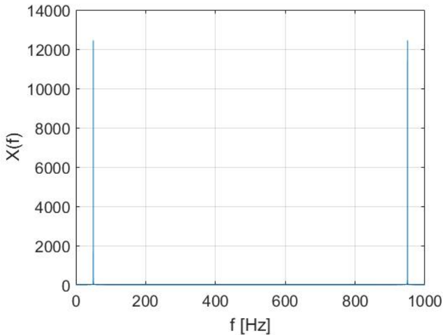
Fig. 8.89: 信号的频谱
