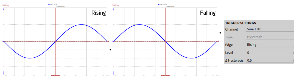
Fig. 8.39: 上升沿 (左) 和下降沿 (右) 触发
