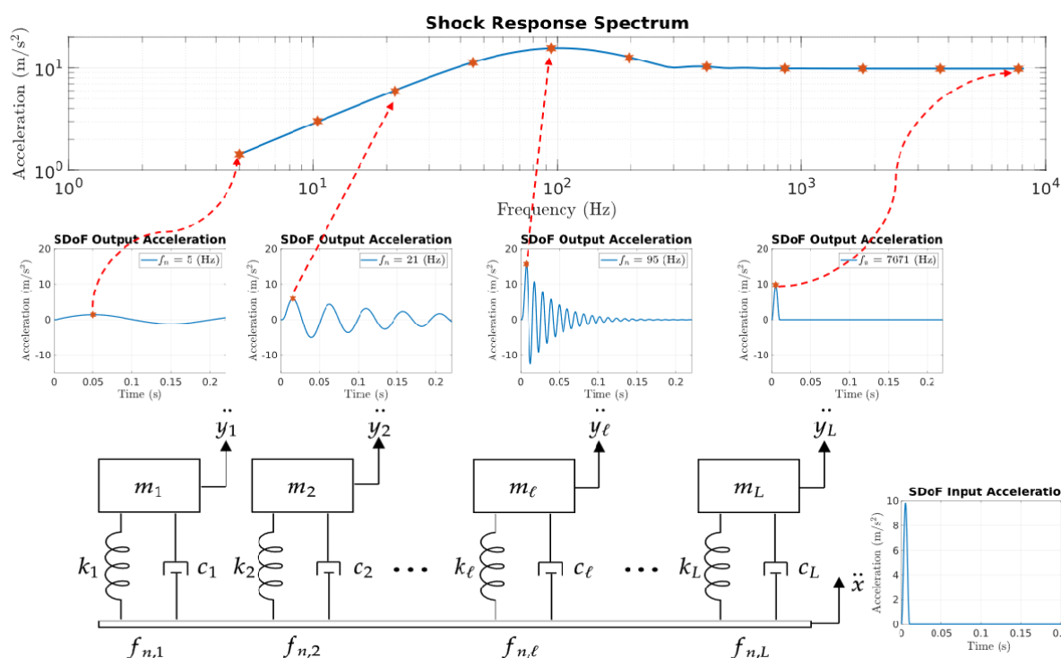
Fig. 7.150: 计算冲击响应谱的示意程序
