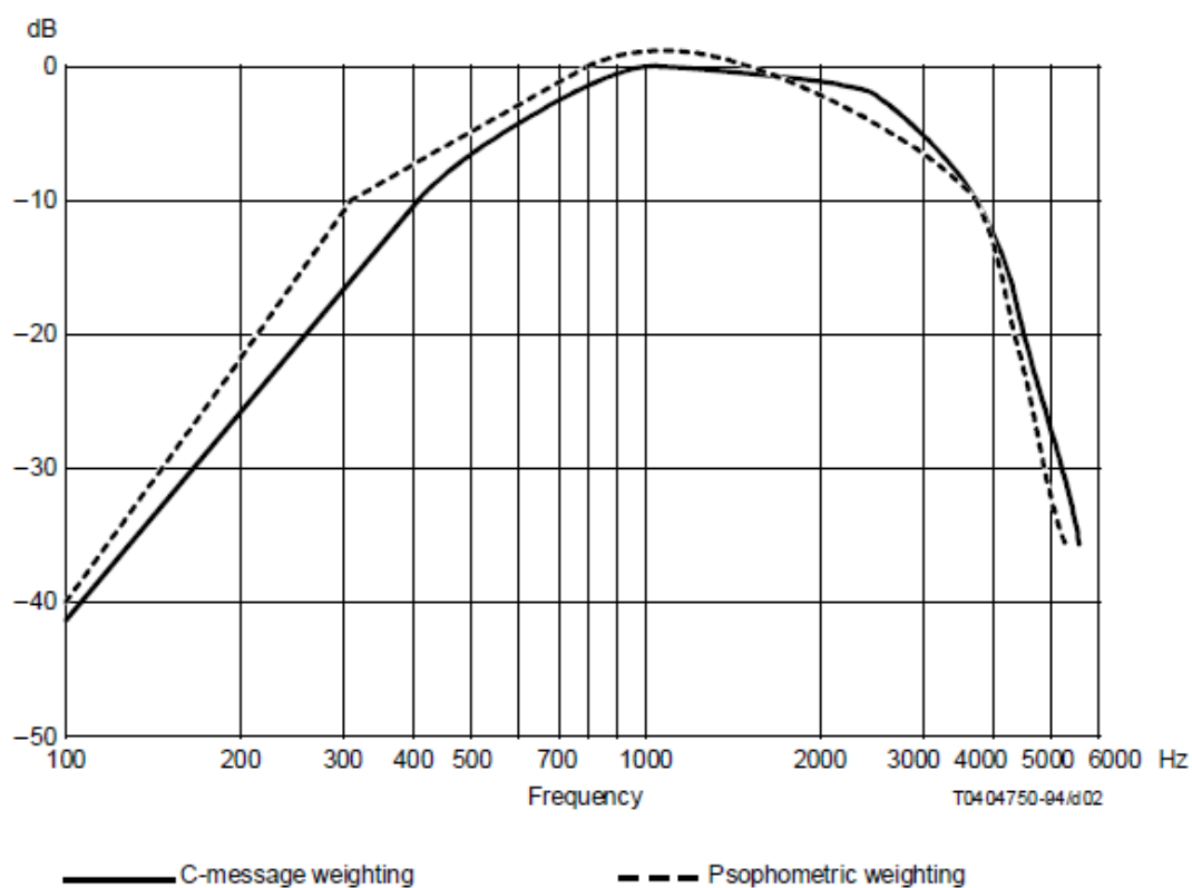
Fig. 7.147: Psophometric 与 C-message 加权之间的比较
