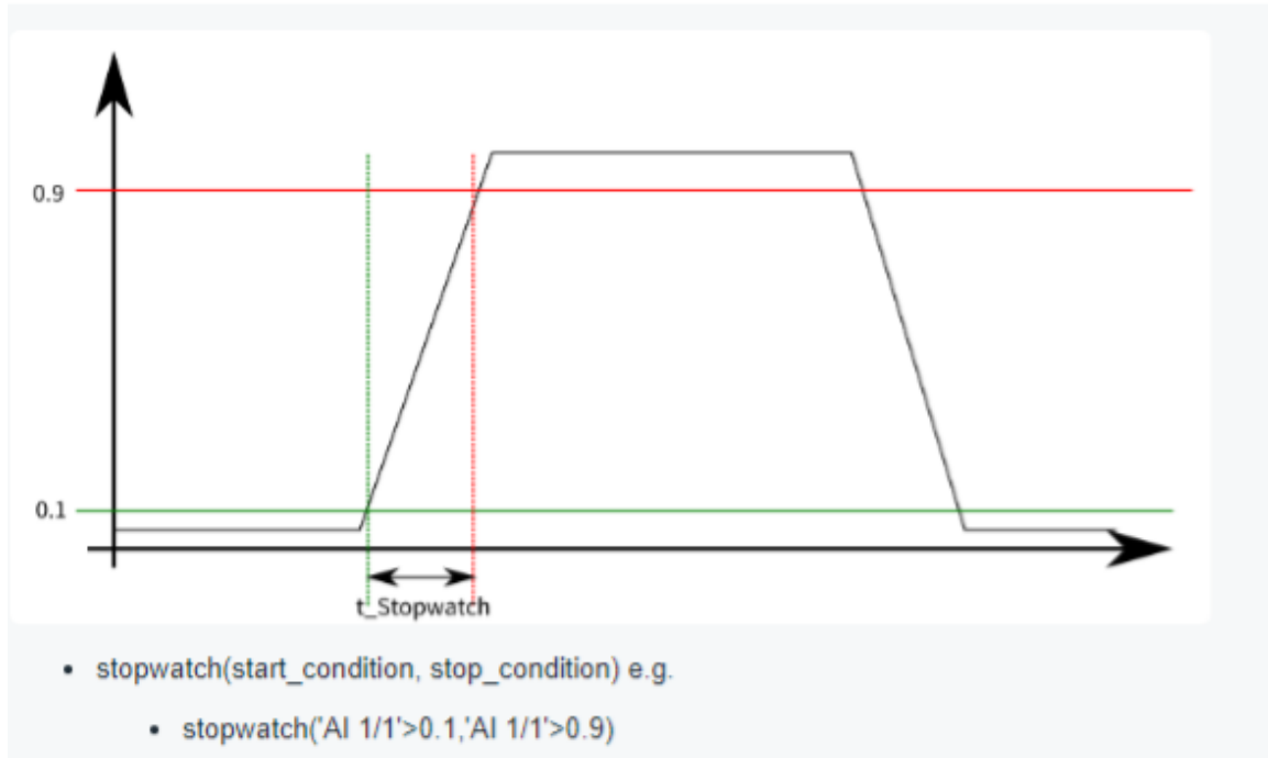
Fig. 7.63: 秒表计原理示意图
