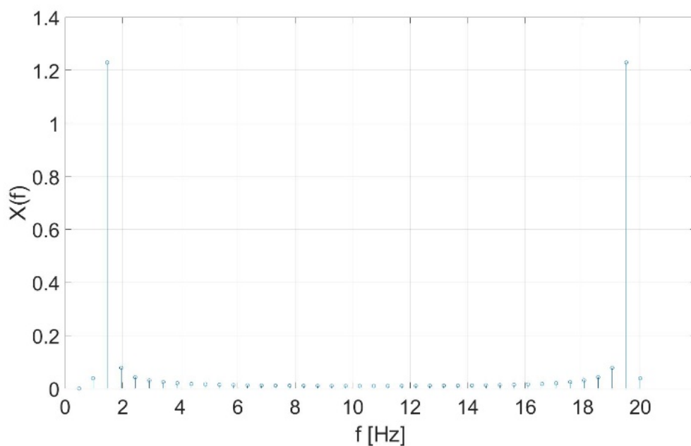
Fig. 8.81: 信号 1 的频谱, 无零填充
