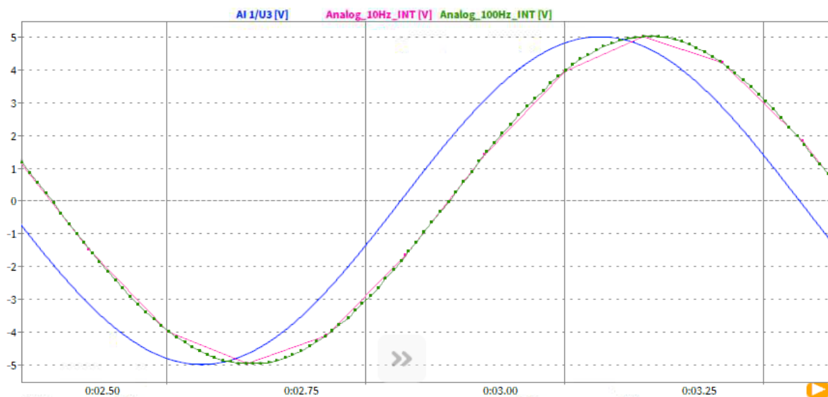
Fig. 7.216: 蓝色曲线为模拟信号输入，绿色曲线为 70ms 延迟下的 CAN 输出曲线
