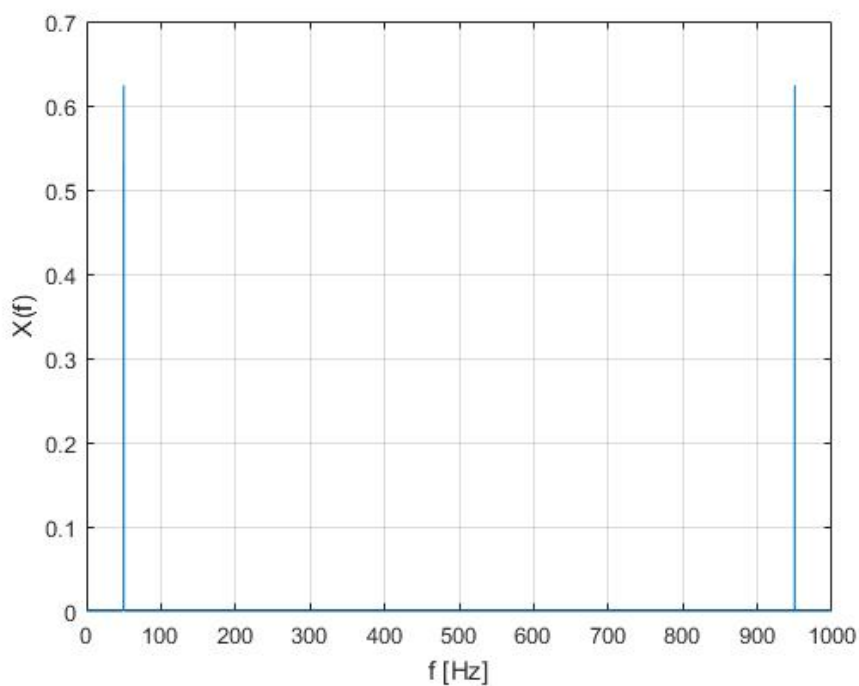
Fig. 8.94: x(t)_{\text{win}} 频谱图 (除以 FFT 长度之后)
