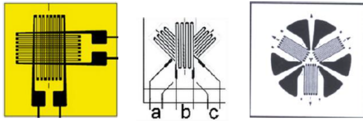
Fig. 7.116: 应变花类型草图
