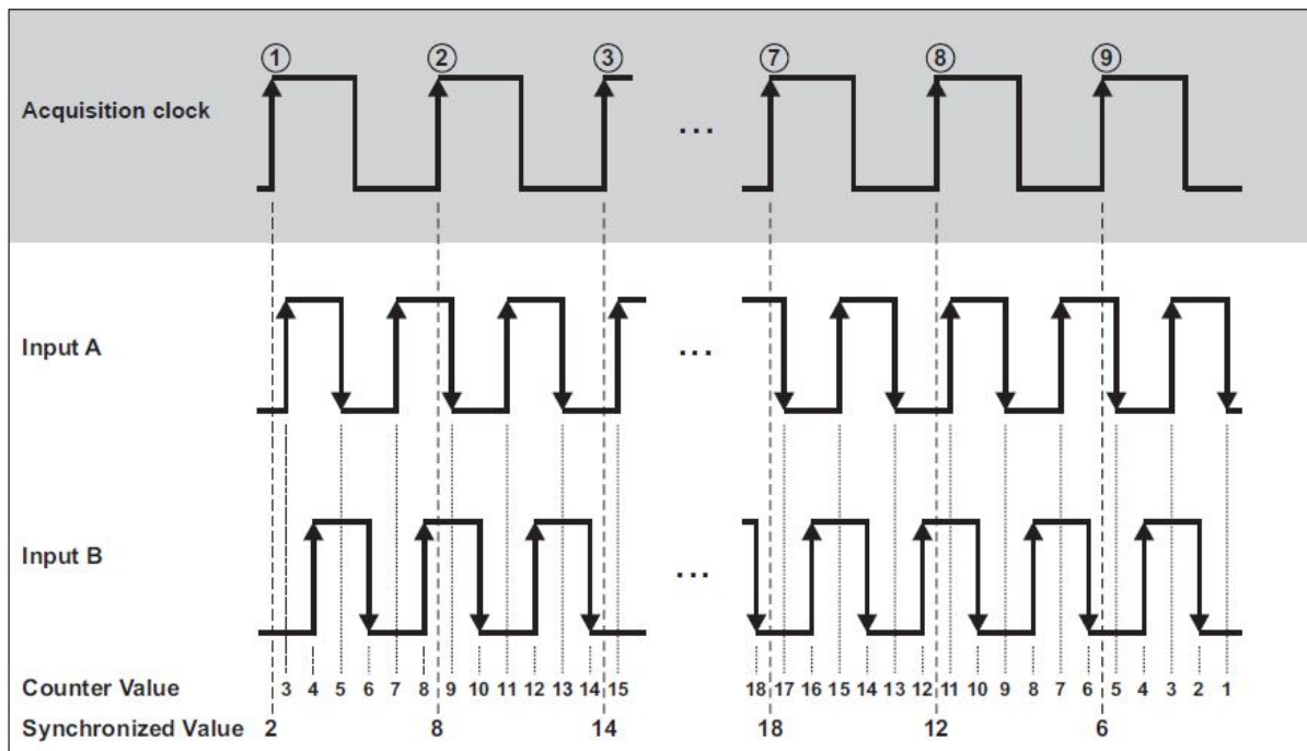
Fig. 7.188: 90 度正交编码器 X4 模式
