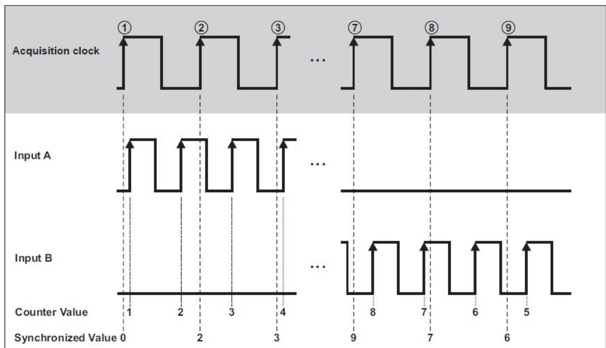
Fig. 7.190: A 上升/B 下降编码器
