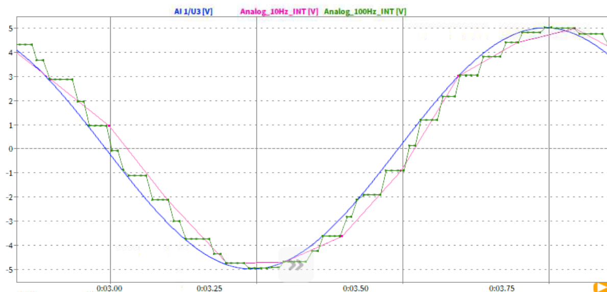
Fig. 7.217: 蓝色曲线为模拟信号输入，绿色曲线为 10ms 延迟下的 CAN 输出曲线
