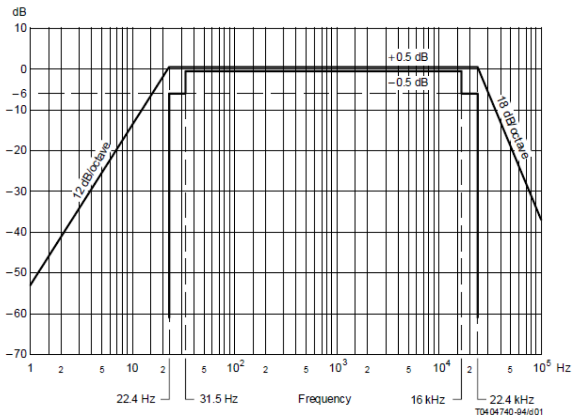
Fig. 7.146: unweighted 测量的频率响应特性
