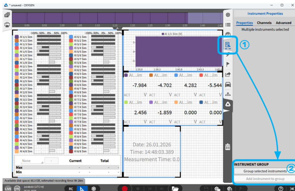
Fig. 8.5: 乐器的分组
