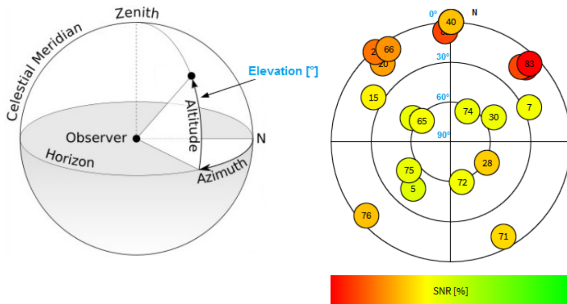
Fig. 8.110: 卫星图解释
