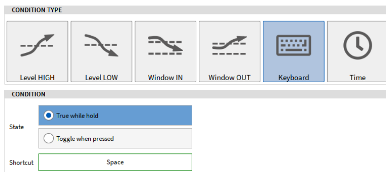
Fig. 9.38: 空格键触发
