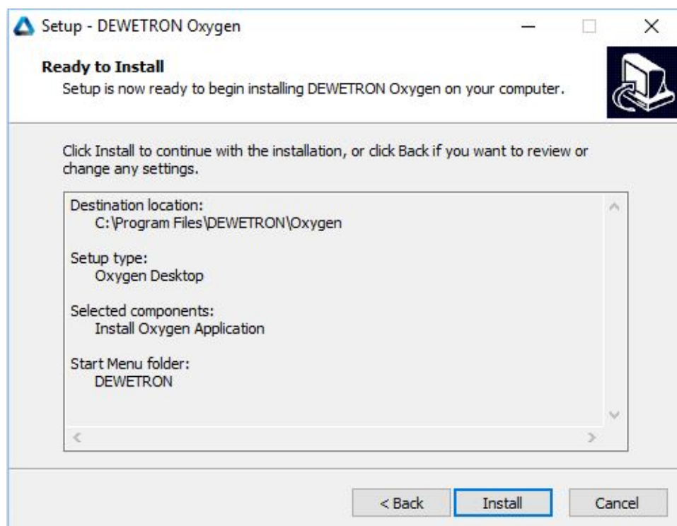
Fig. 2.5: 准备好安装
