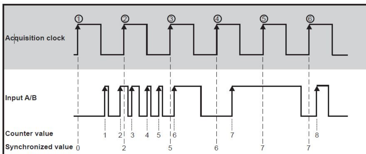
Fig. 7.182: 时间计数
