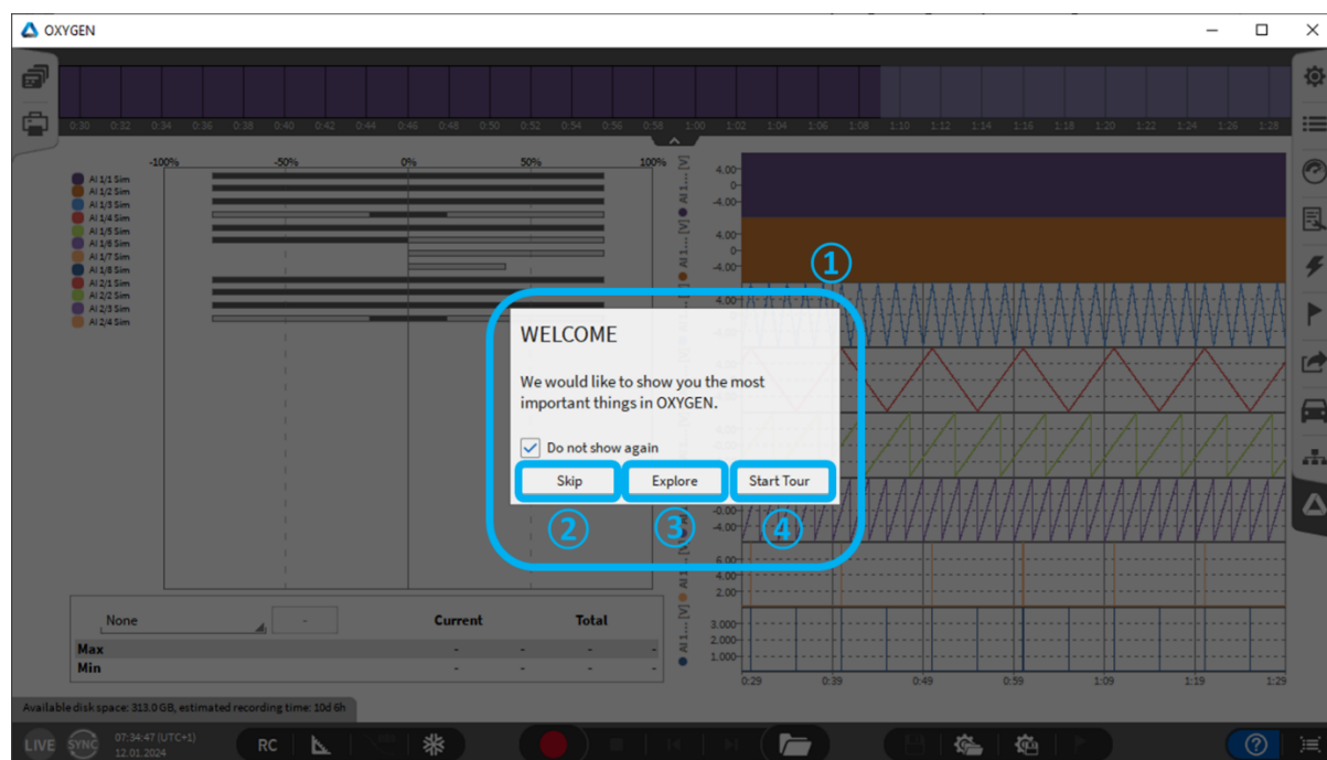
Fig. 3.1: 欢迎导览
