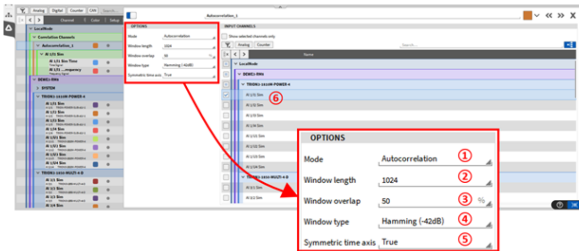
Fig. 7.105: 自相关-设置
