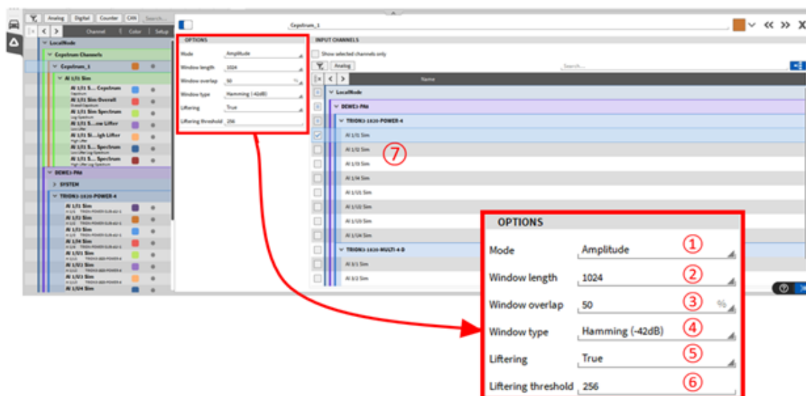
Fig. 7.103: 倒频谱设置
