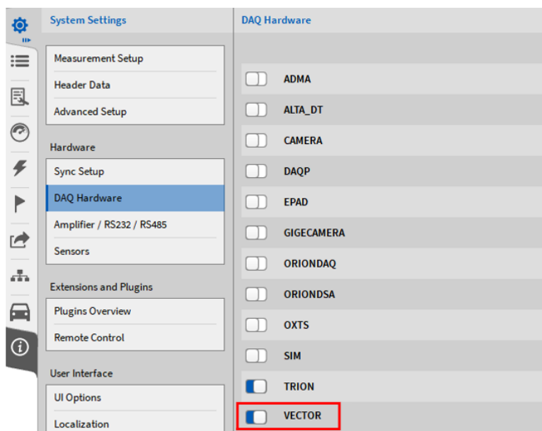
Fig. 4.49: 激活 CAN-FD
