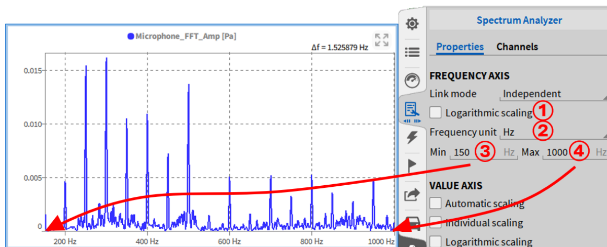
Fig. 8.54: 频率轴设置
