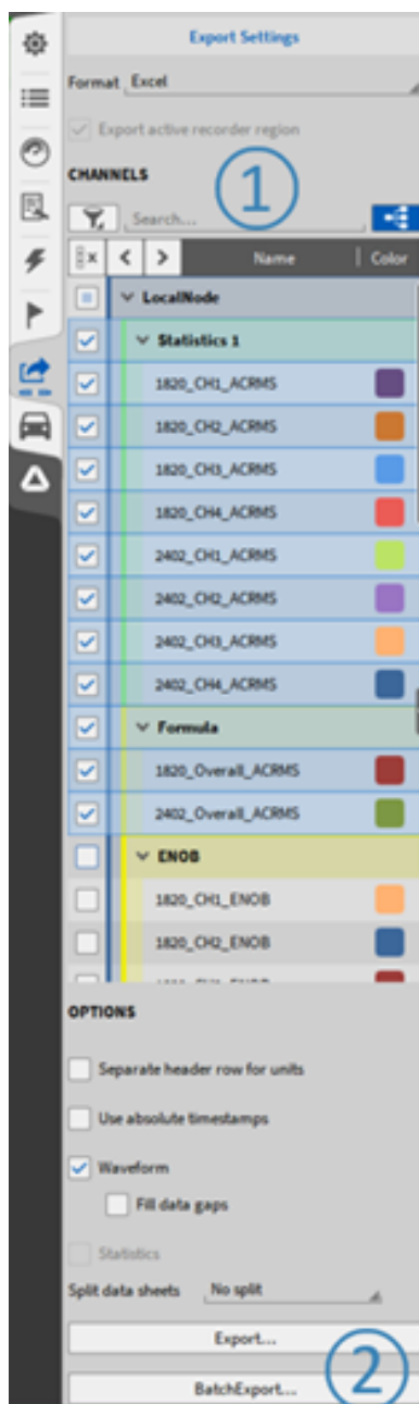
Fig. 11.22: 导出菜单
