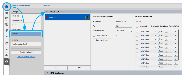
Fig. 5.46: MODBUS 服务器
