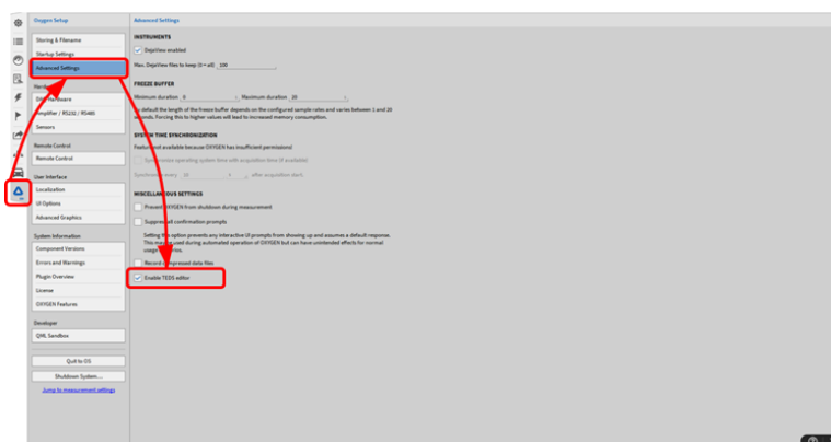
Fig. 7.222: TEDS 信息
