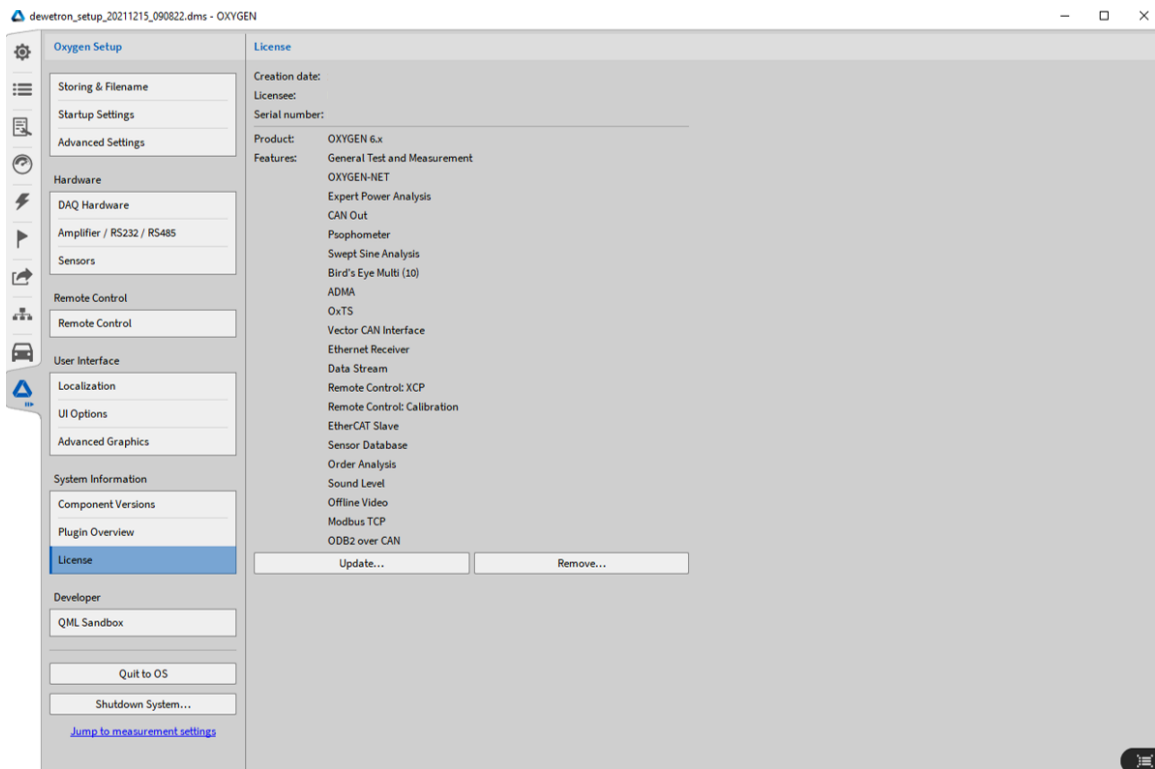
Fig. 6.31: 授权概览
