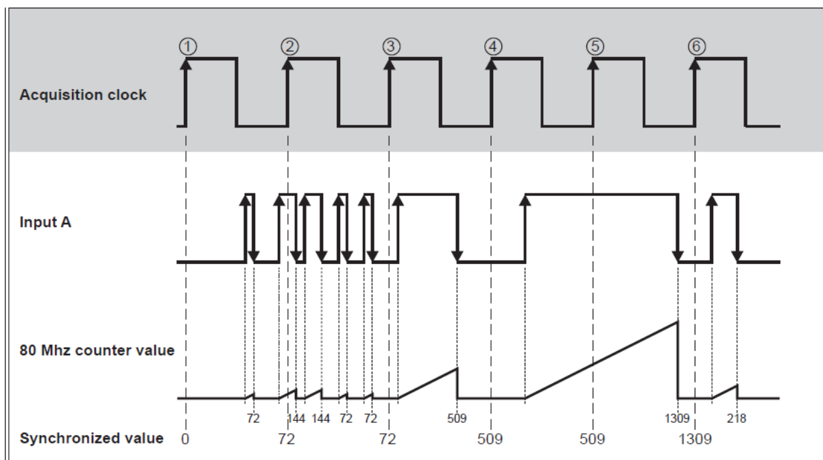
Fig. 7.185: 脉冲宽度测量
