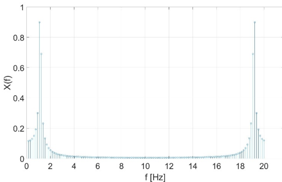
Fig. 8.87: 信号 2 的频谱, 无零填充
