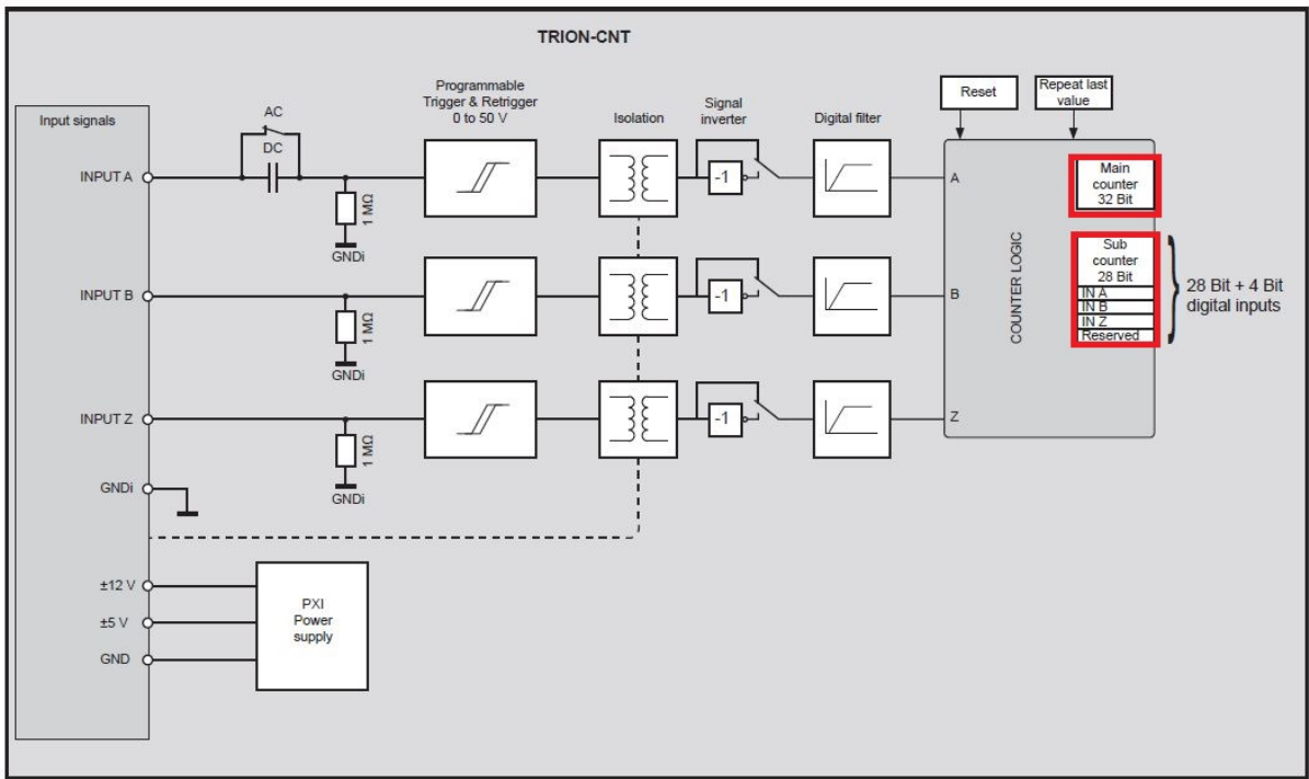
Fig. 7.192: TRION-CNT 模块内部电路
