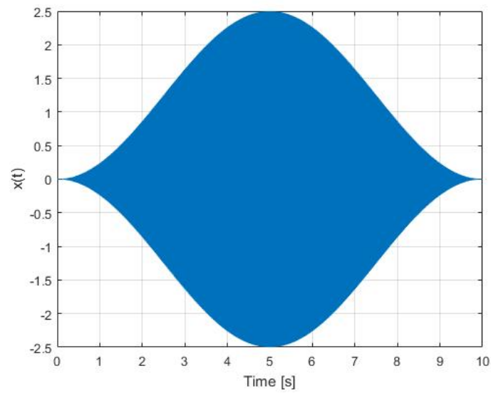
Fig. 8.92: x(t)_{\text{win}} 时域波形; 添加了汉宁窗
