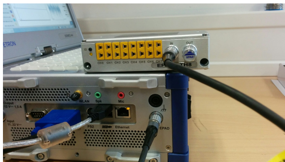
Fig. 4.21: EPAD 模块接口
