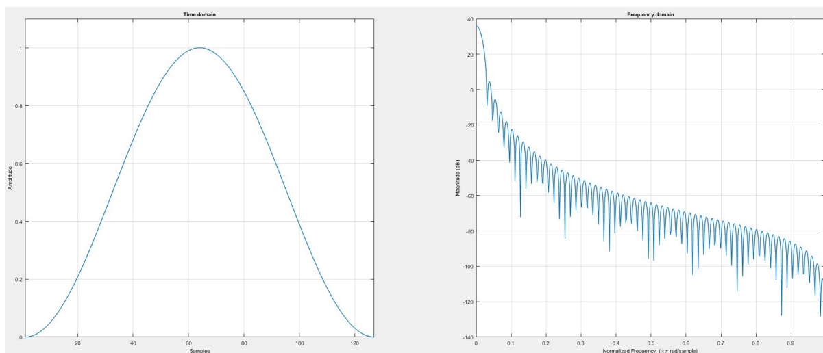
Fig. 8.57: 汉宁窗频域和时域特征图 (N=128)
