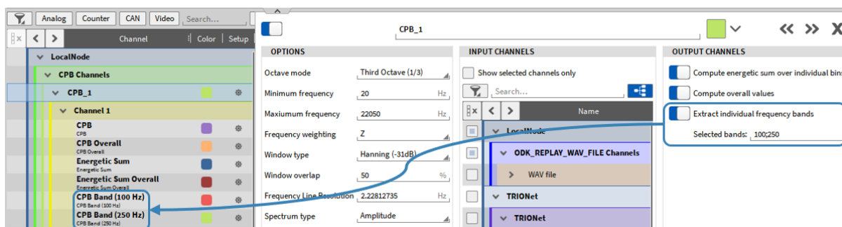
Fig. 7.130: 使用 CPB 倍频程分析提取 100Hz 和 250Hz 频段信号
