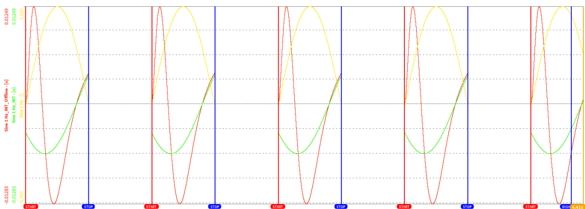
Fig. 7.179: 触发记录波形在线滤波器积分计算和离线滤波器积分计算的区别
