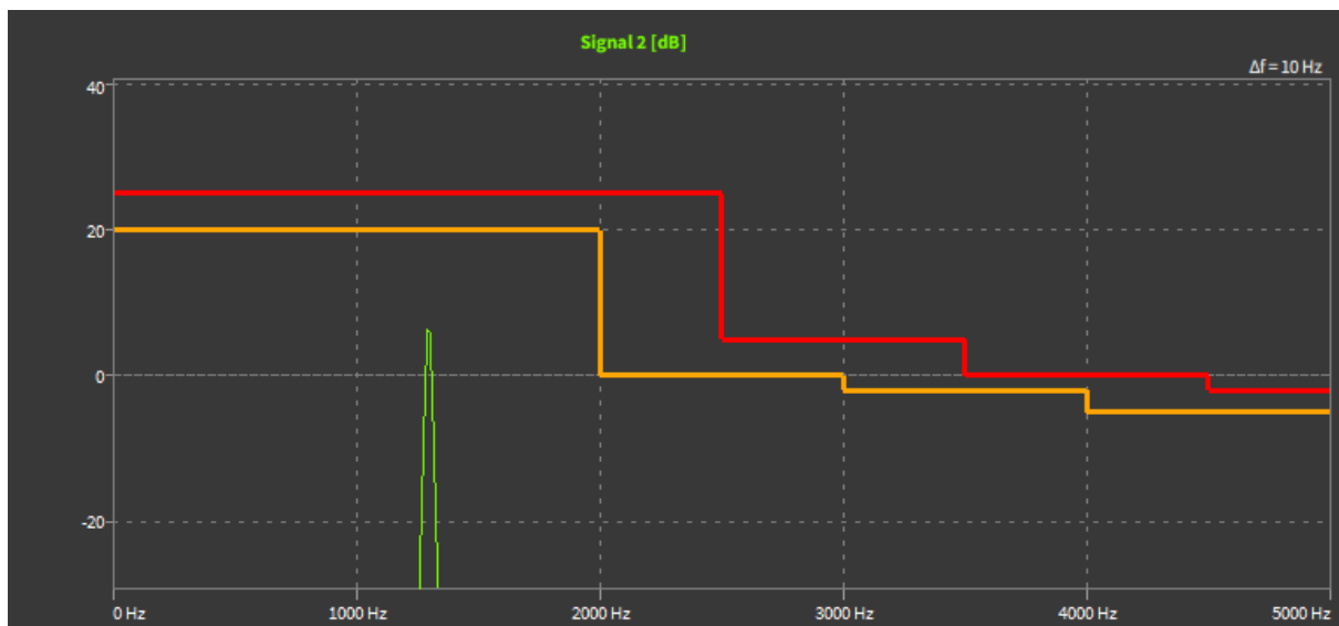
Fig. 8.74: 未超限的参考曲线
