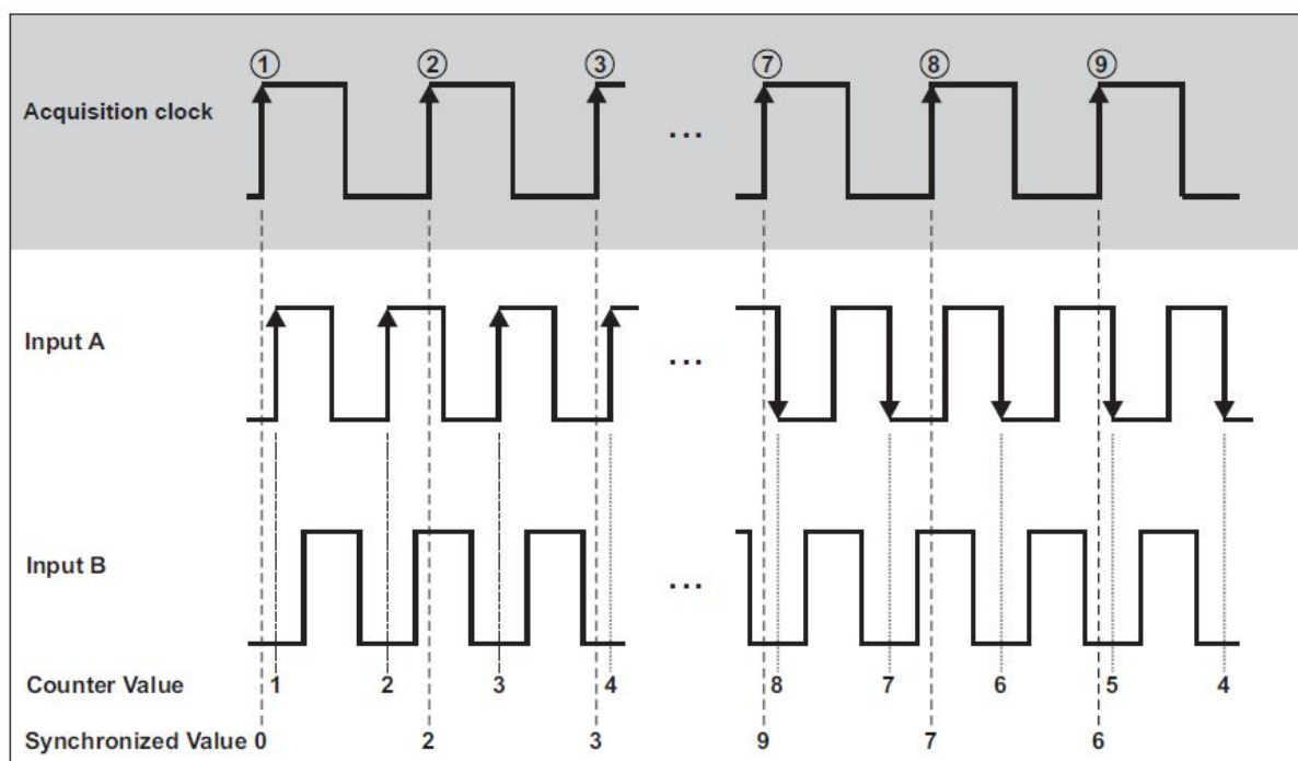
Fig. 7.186: 90 度正交编码器 X1 模式
