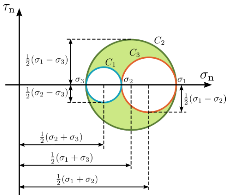
Fig. 7.115: 莫尔圆
