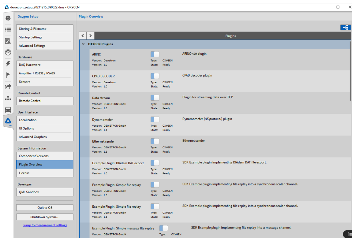
Fig. 6.30: 插件概览
