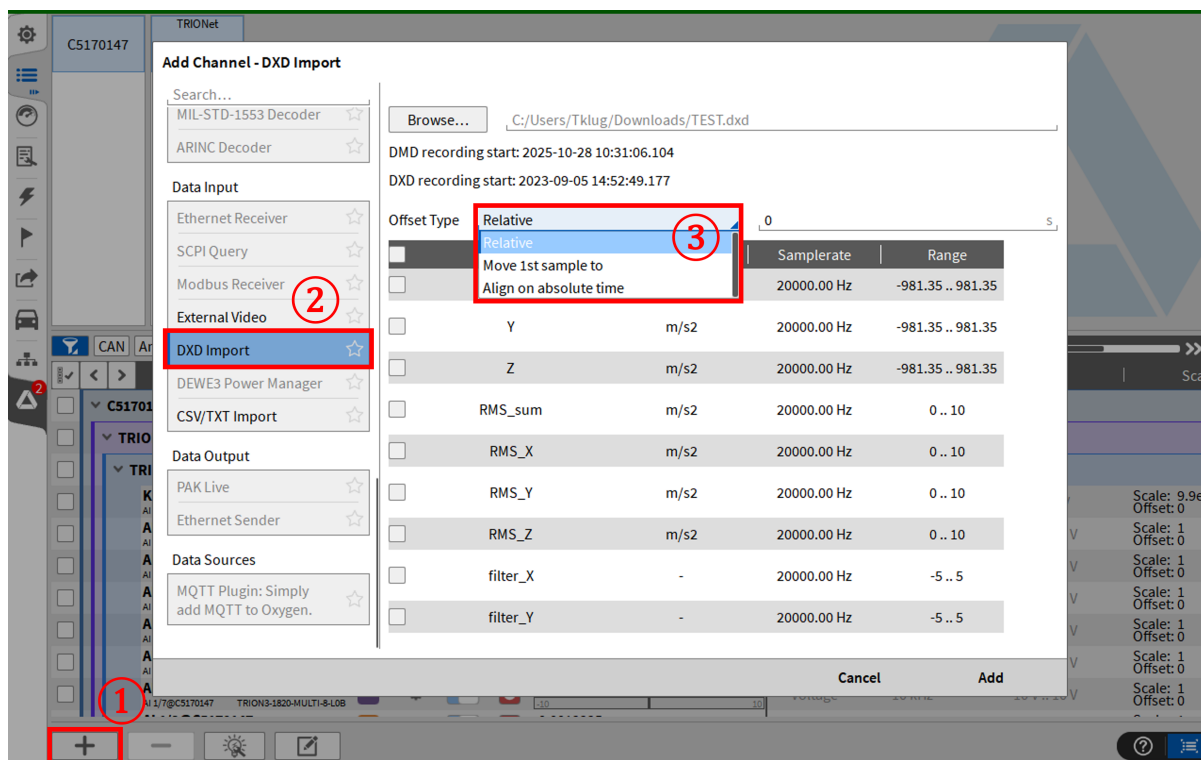
Fig. 7.171: DXD 导入
