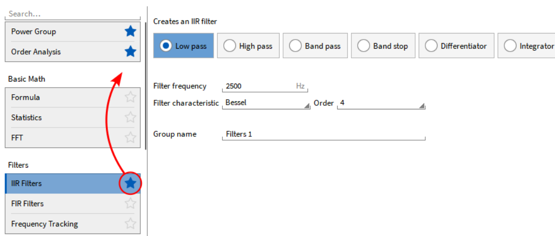
Fig. 7.54: 添加收藏
