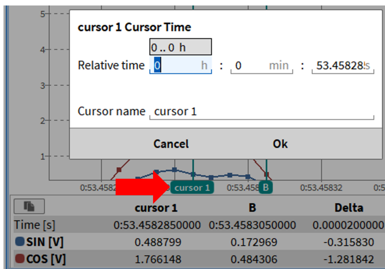
Fig. 8.32: 重命名光标
