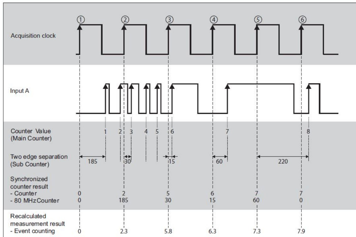
Fig. 7.184: 频率测试
