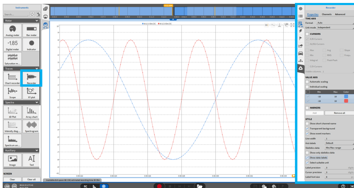
Fig. 8.20: 波形记录仪
