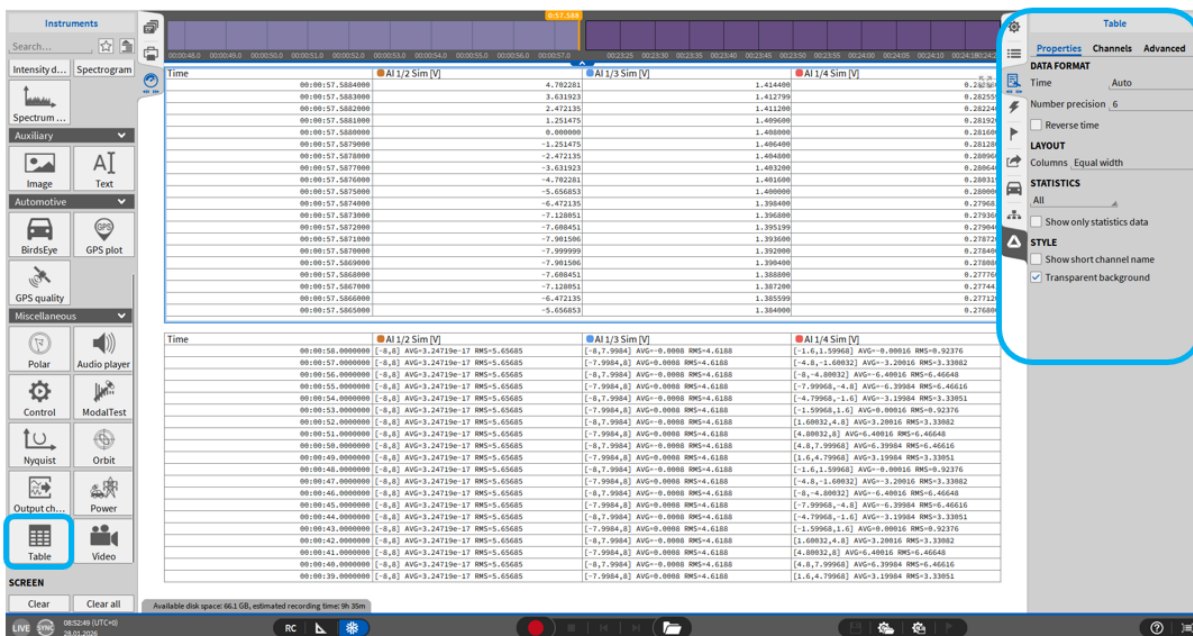
Fig. 8.132: 表格-总览
