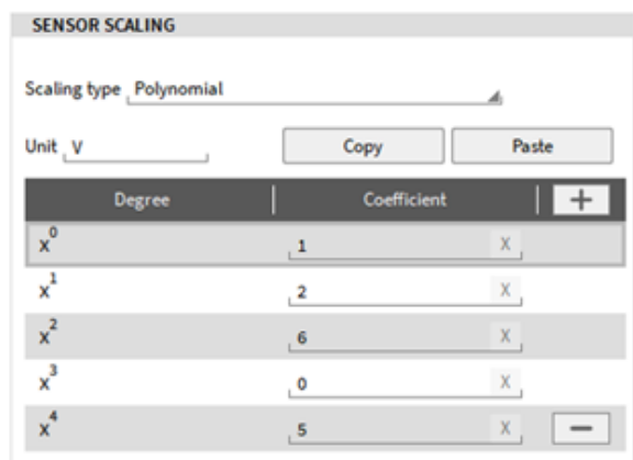
Fig. 7.43: 多项式系数
