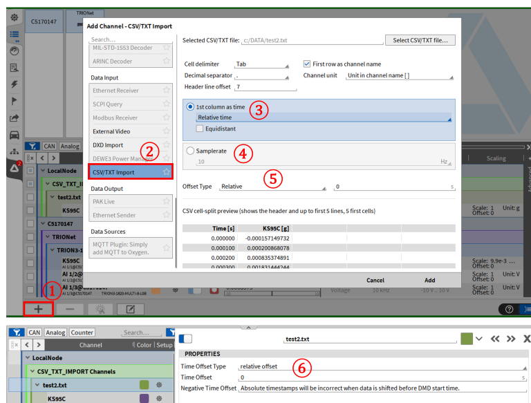
Fig. 7.172: CSV/TXT 导入
