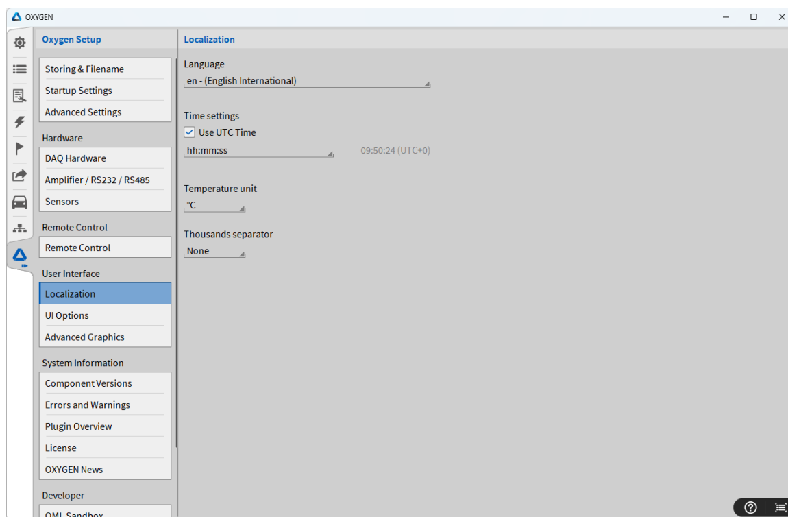
Fig. 6.25: 本地化-设置
