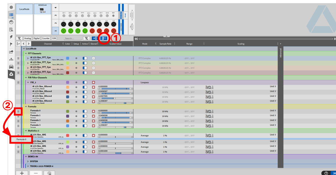
Fig. 7.3: 通道排序
