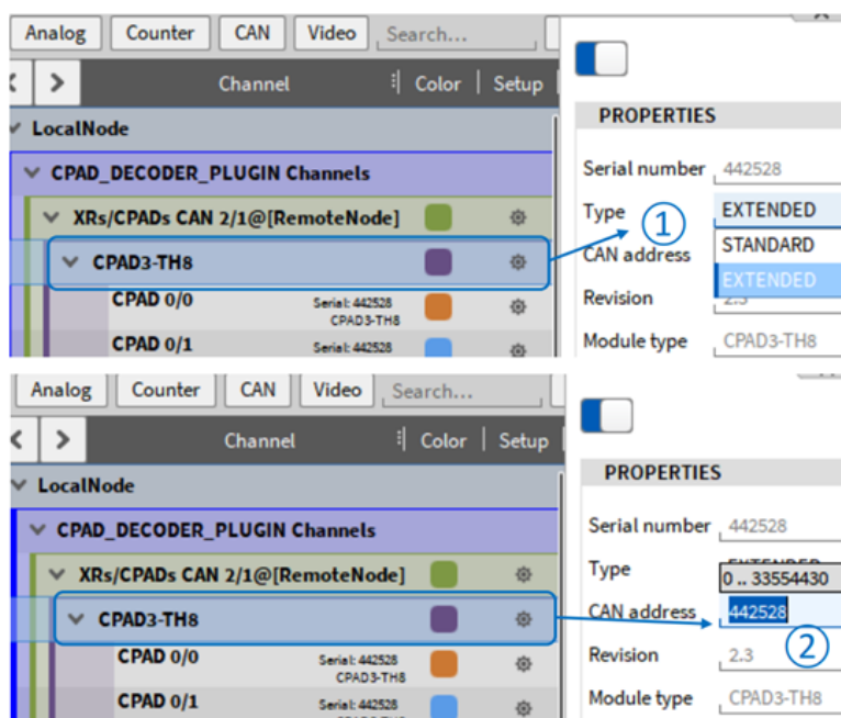
Fig. 4.35: CPAD 属性
