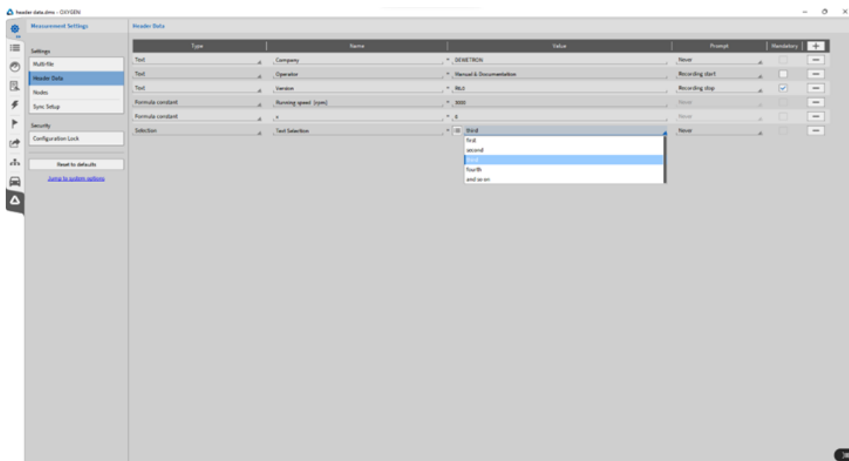
Fig. 5.20: 数据头设置
