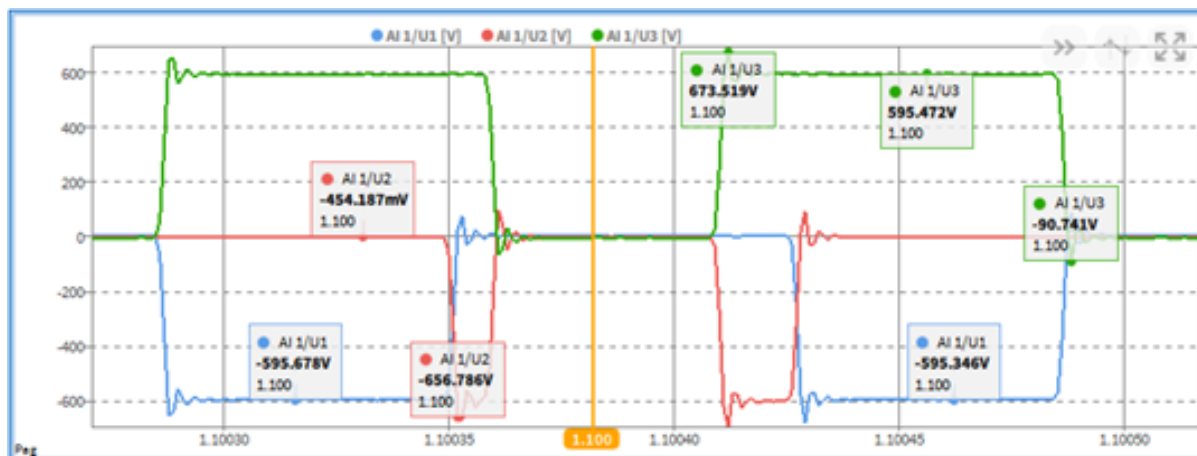
Fig. 3.9: 激活标签
