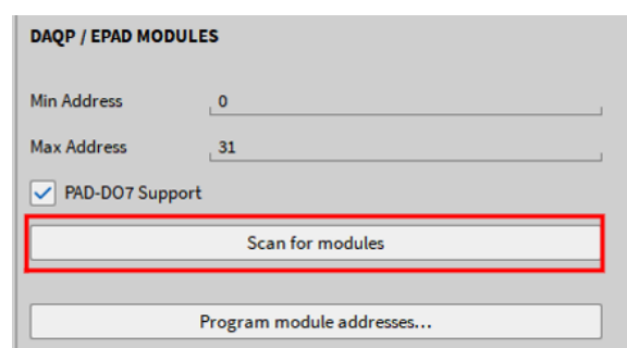
Fig. 4.24: 搜索按钮
