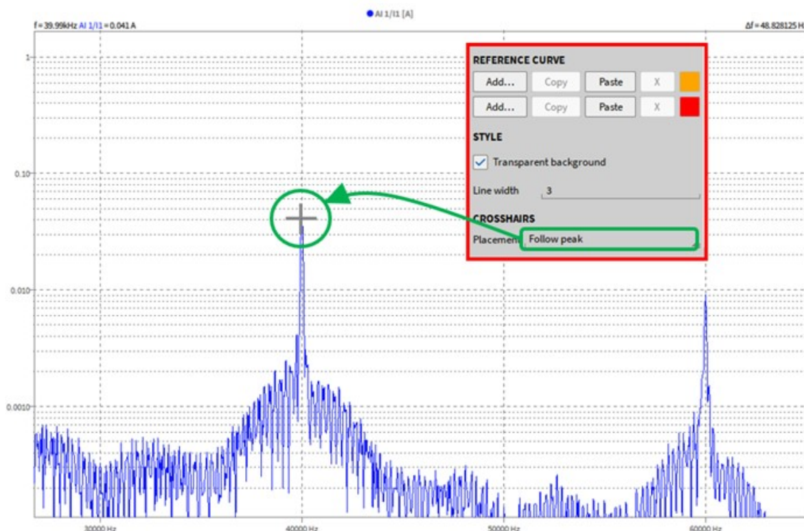
Fig. 8.78: 峰值追踪
