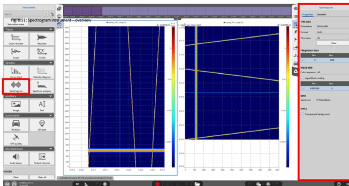
Fig. 8.51: 色谱图-总览
