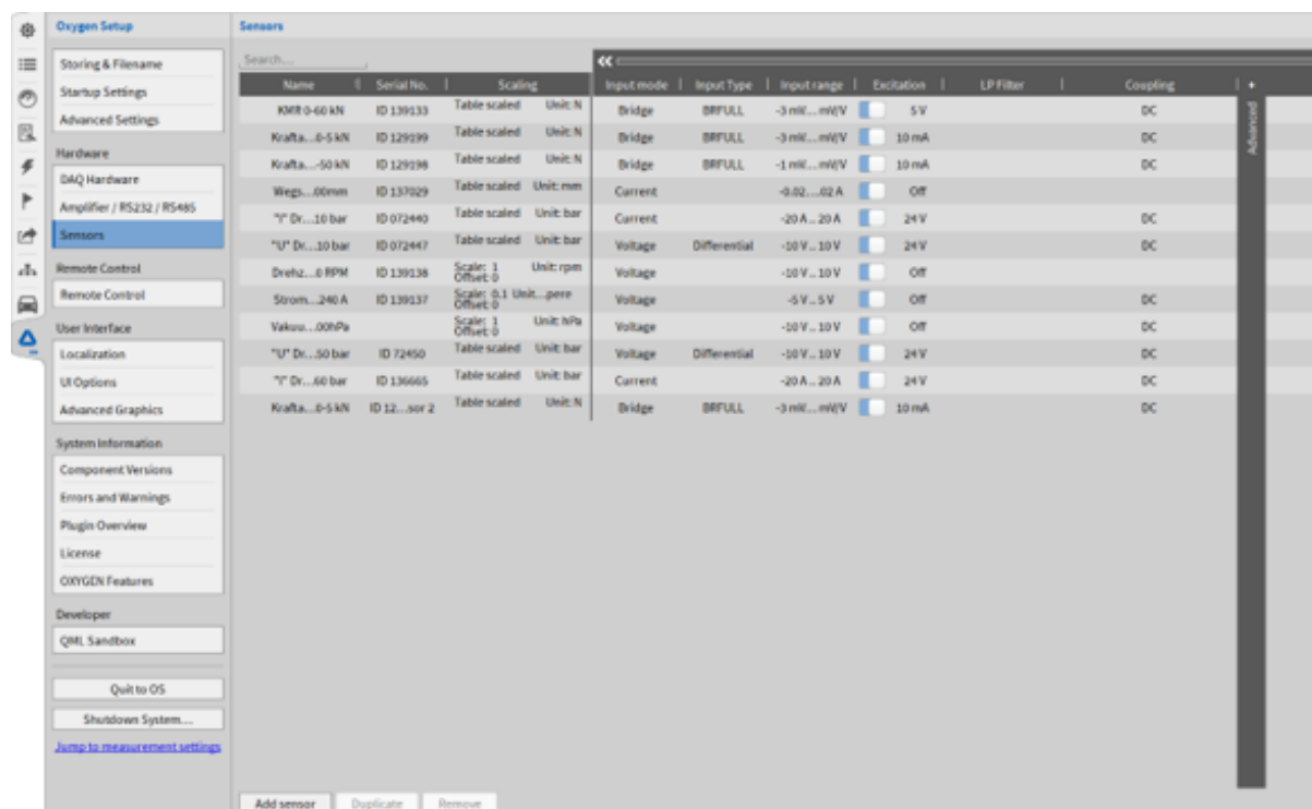
Fig. 6.11: 传感器库
