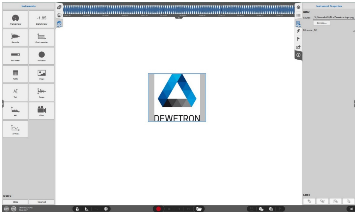
Fig. 8.101: 图片 - 总览
