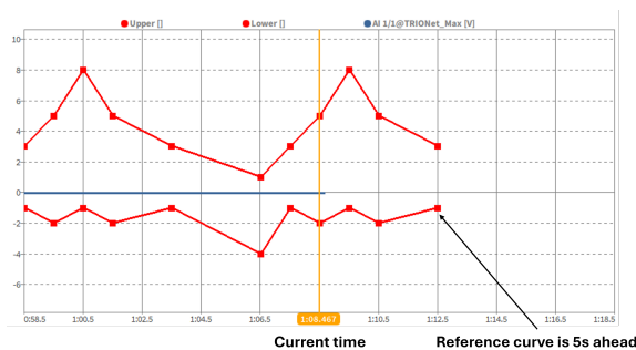
Fig. 7.120: 具有 5 s 预填充时间（Fill ahead time）的上限和下限时间参考曲线示例
