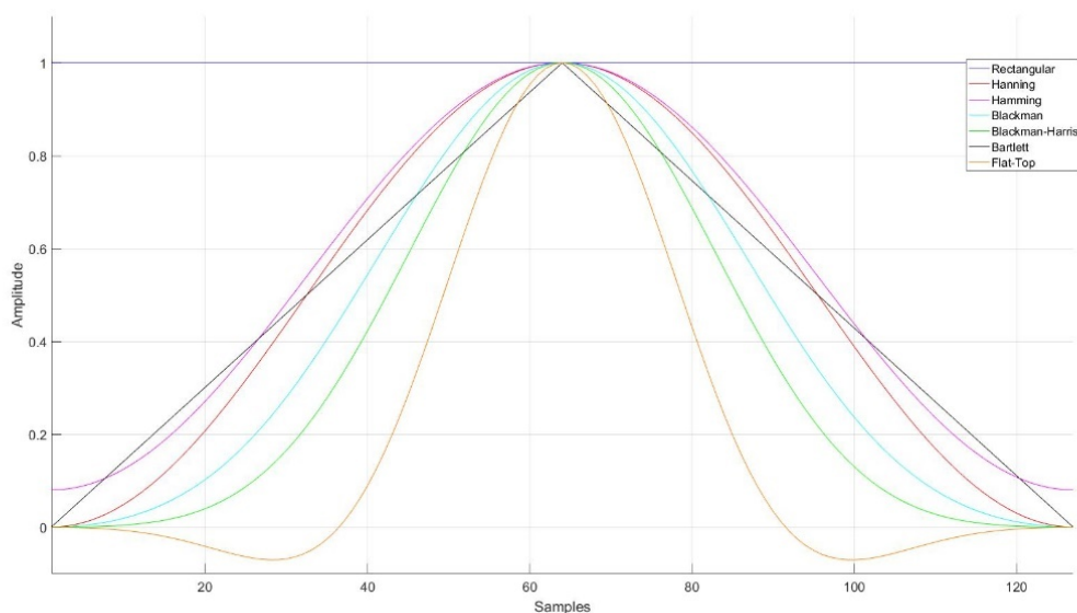
Fig. 8.63: 不同窗函数的时域图 (N = 128)
