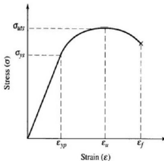
Fig. 7.117: 应变-应力曲线
