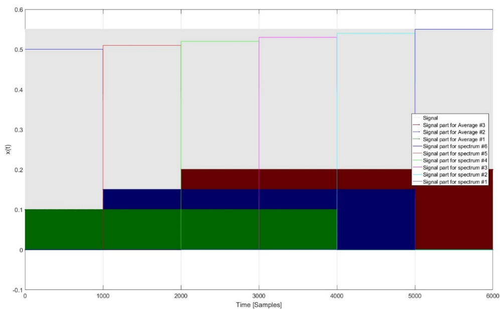
Fig. 8.98: 期图的时间信号分解, 平均谱为 4, 重叠 0%
