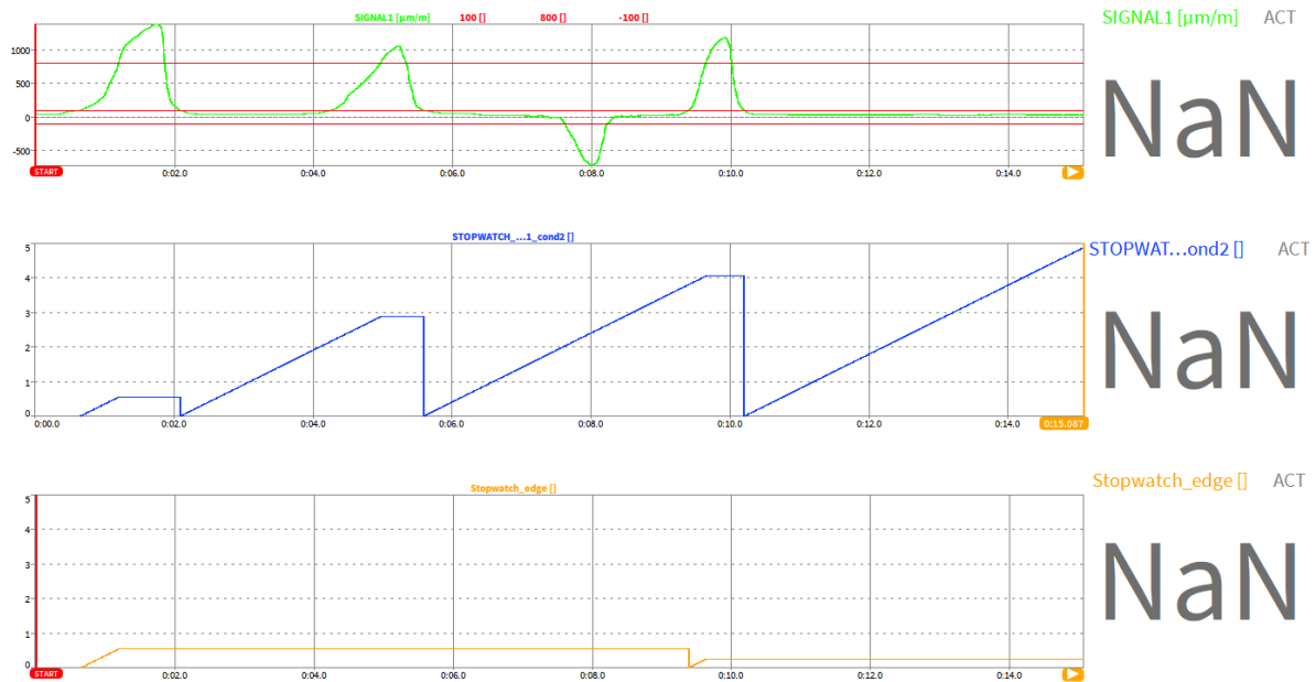
Abb. 7.73: Kombination der edge und stopwatch Funktion
