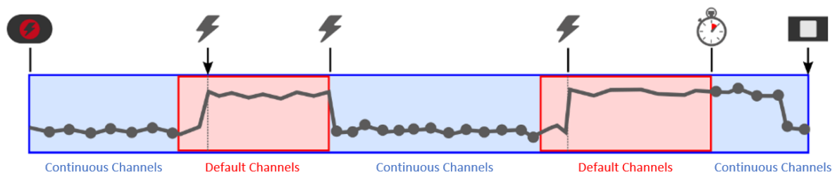
Abb. 9.44: Darstellung der Speicherung von Continuous und Default Kanälen
