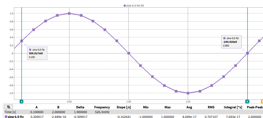
Abb. 8.33: 0.5 Hz Sinuskurve in einem Rekorder; Cursor A @ 0.1s und Cursor B @ 2.0s
