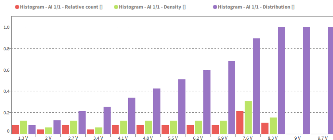
Abb. 7.124: Beispieldarstellung eines Histogramms für Relative Anzahl, Dichte und Verteilung
