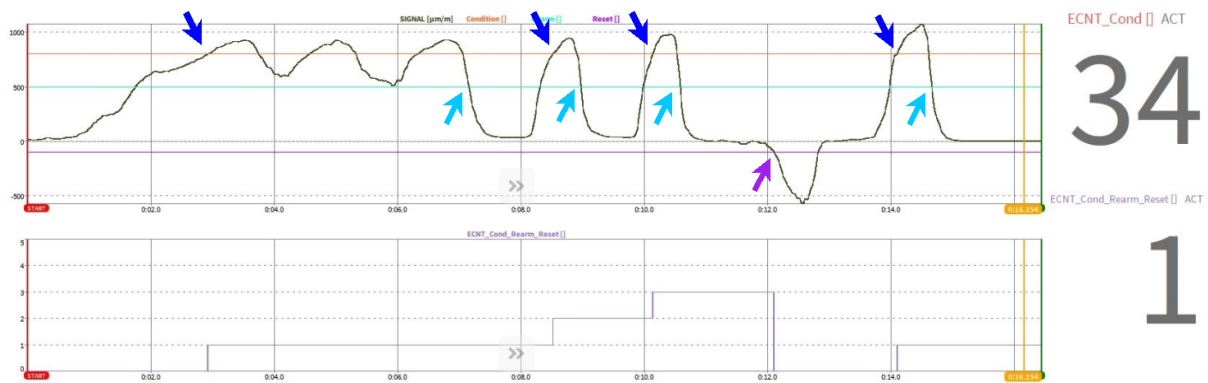
Abb. 7.59: ECNT-Funktion mit Bedingung , Rearm und Reset
