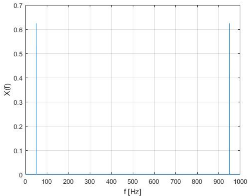
Abb. 8.92: Einseitiges Spektrum X(f)_{\text{win}} mit dem Faktor 2 multipliziert
