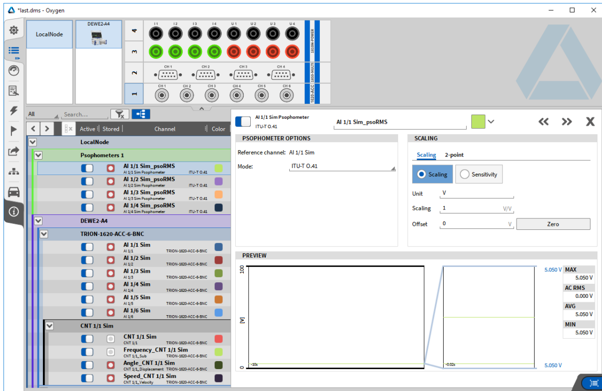
Abb. 7.141: Kanaleinstellungen für einen Psophometer-Berechnungskanal
