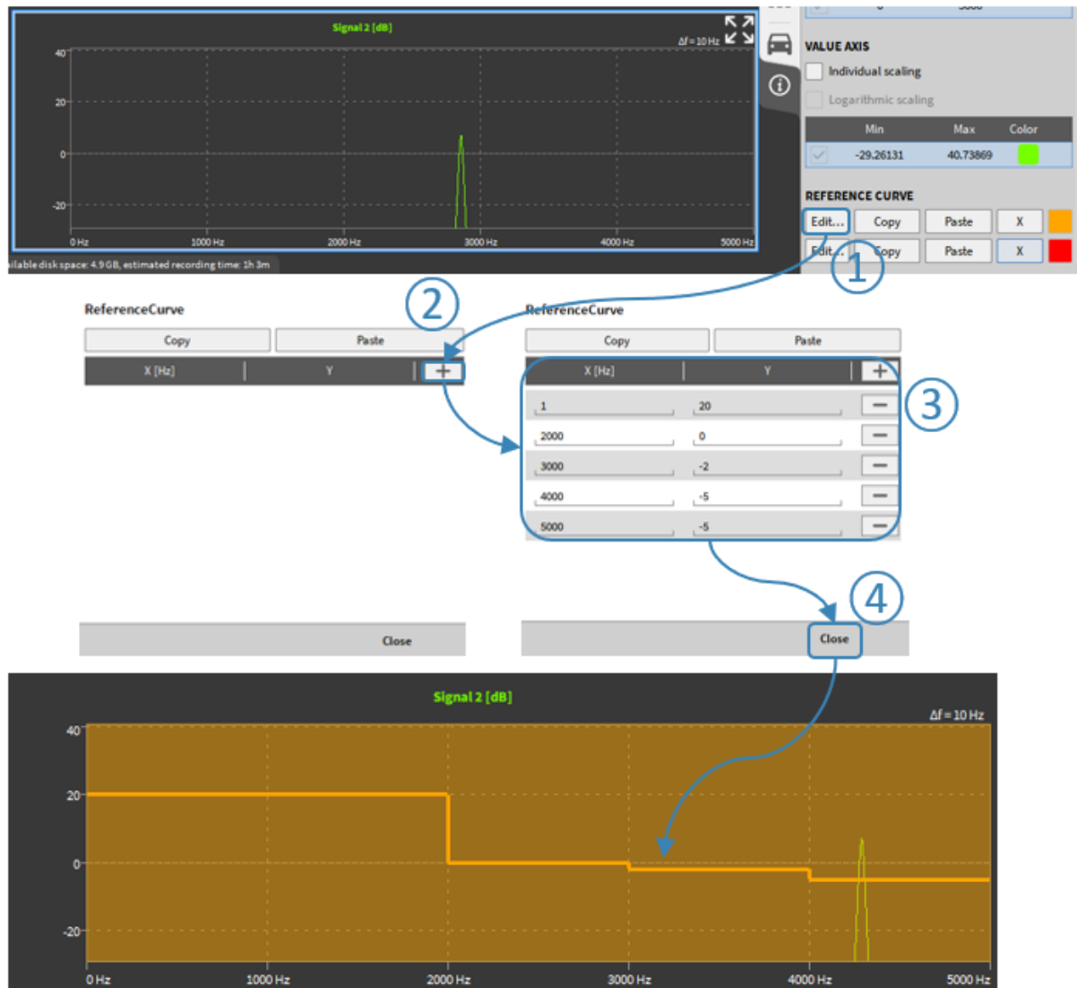
Abb. 8.68: Erstellung einer orangen Referenzkurve
