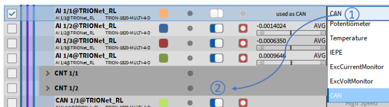
Abb. 7.204: CAN-Ports eines TRION-MULTI-Moduls
