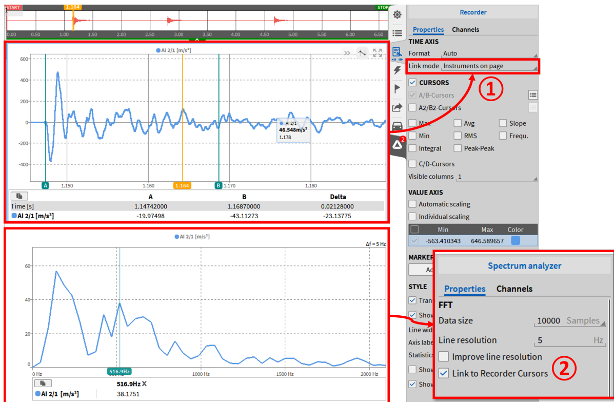
Abb. 8.77: FFT-Berechnung auf Basis von Rekorderauswahl
