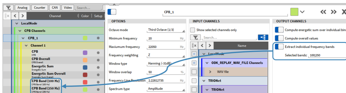
Abb. 7.130: CPB Analyse mit extrahiertem 100 Hz und 250 Hz Bin
