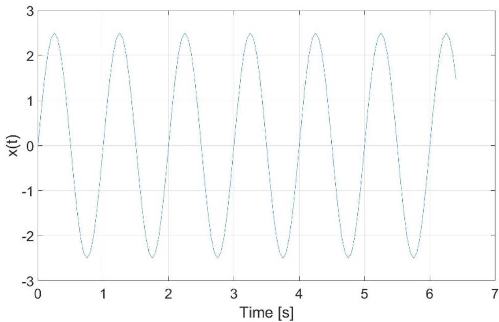
Abb. 8.84: Signal 2 im Zeitbereich, 6,4s (128 Samples)
