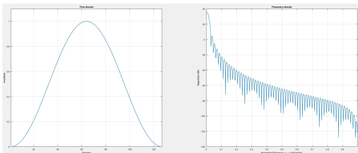
Abb. 8.57: Hanning-Fenster in Zeit- und Frequenzbereich (N = 128)
