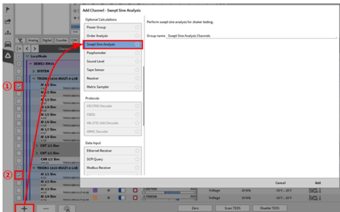
Abb. 7.135: Exemplarischer Aufbau für den Gebrauch des Swept-Sine-Analyse Plugins
