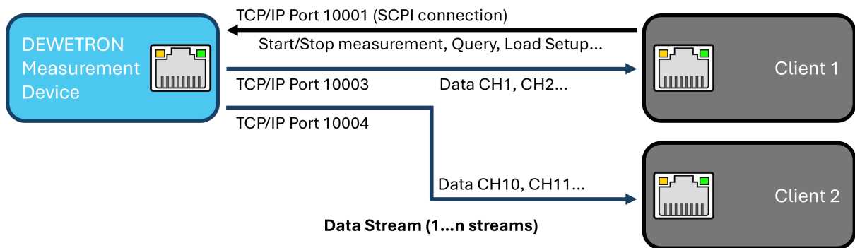
Abb. 6.23: Data Stream Plugin – Übersicht
