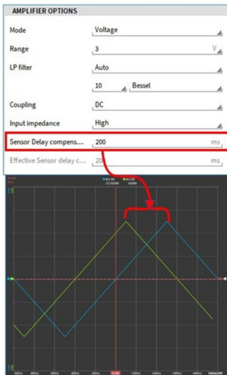
Abb. 7.32: Kompensation der Sensorverzögerung
