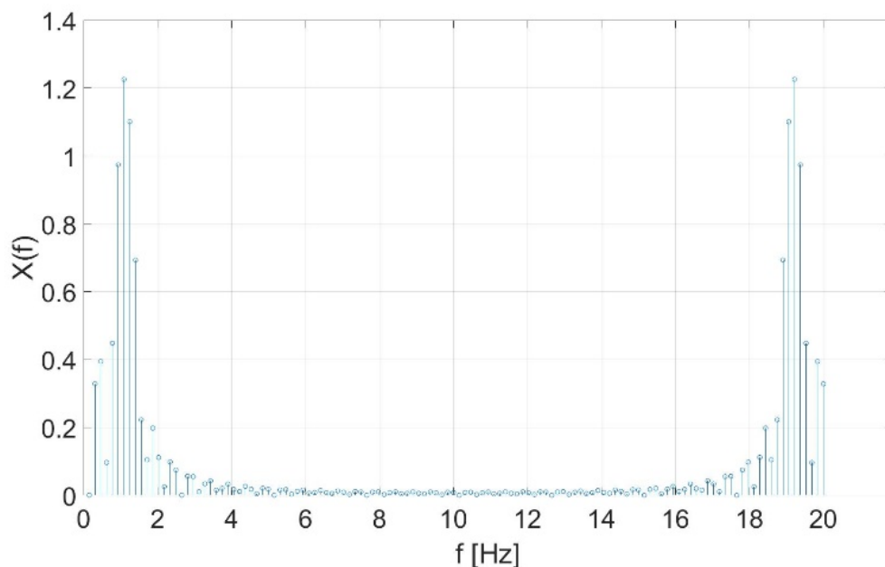
Abb. 8.83: Signal 1 im Frequenzbereich, Zero-Padding auf 128 Samples
