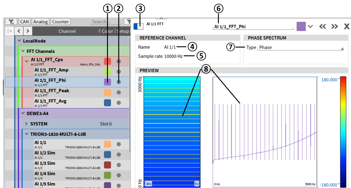
Abb. 7.92: Kanaleinstellungen des Phasenspektrums – Übersicht
