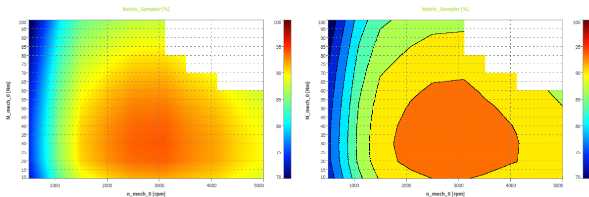
Abb. 8.50: Intensity-Diagramm eines Matrix Samplers ohne (links) und mit Bereichsabgrenzung (rechts, 10 Level)
