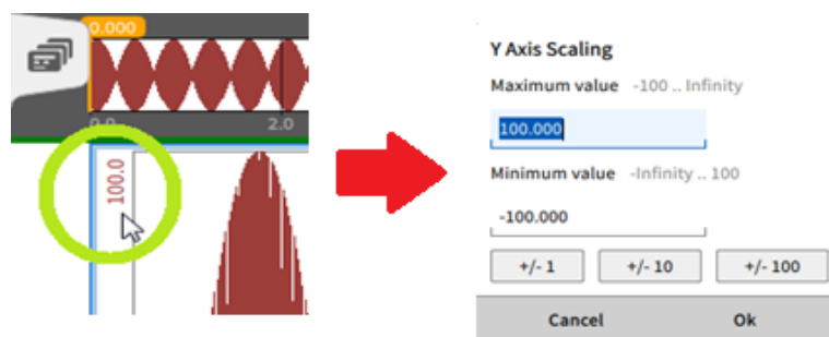
Abb. 8.29: Benutzerdefinierte Y-Achsenkalierung für einen Kanal (Individuelle Skalierung nicht ausgewählt)
