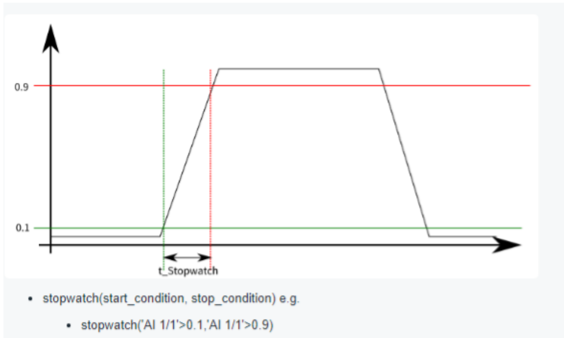
Abb. 7.63: Schematische Erklärung der stopwatch Funktion
