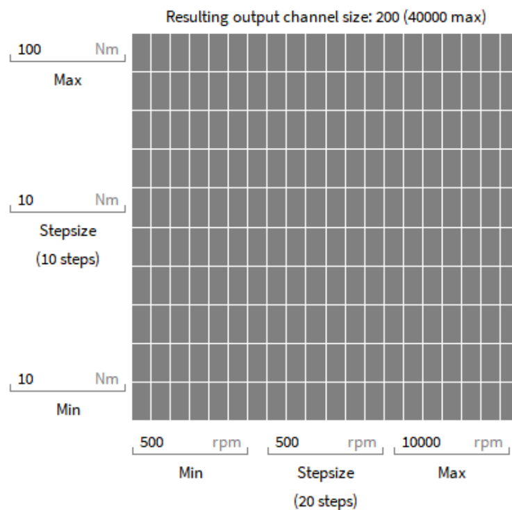
Abb. 7.160: Detail-Ansicht der Vorschau-Matrix in den Einstellungen eines Matrix Sampler Kanals
