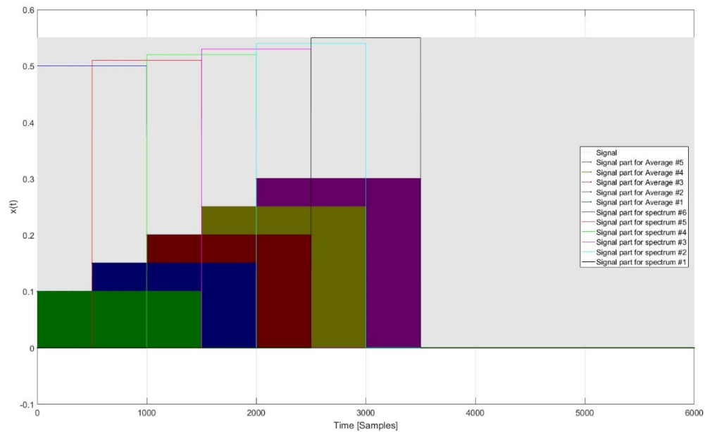
Abb. 8.98: Zerlegung des Signals im Zeitbereich für die Mittelung von 2 Spektren und 50 % Überlappung
