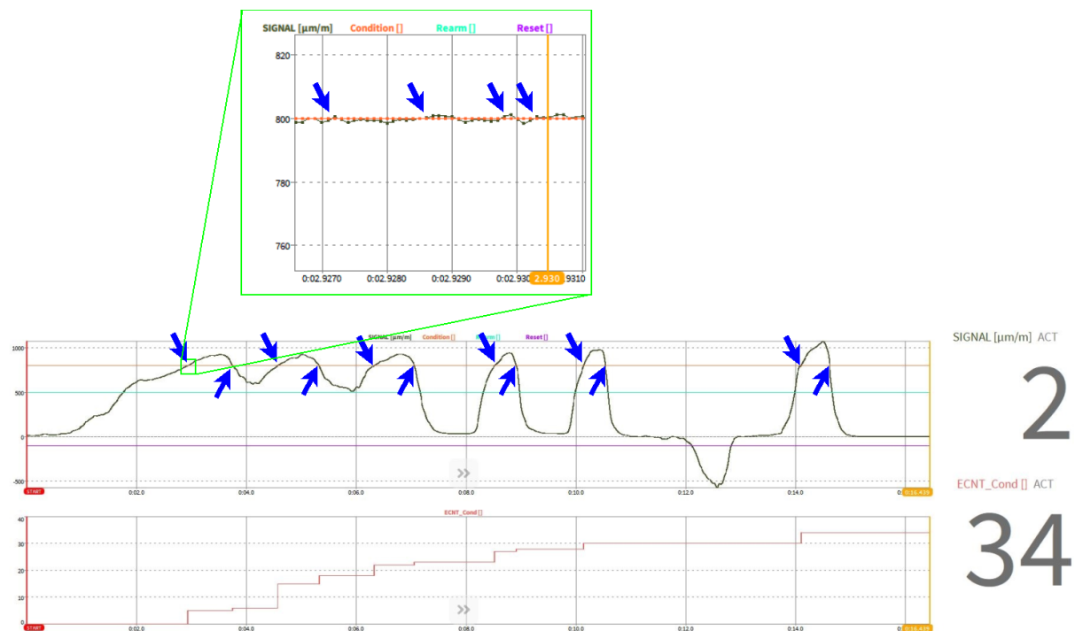
Abb. 7.57: ECNT-Funktion nur mit Bedingung
