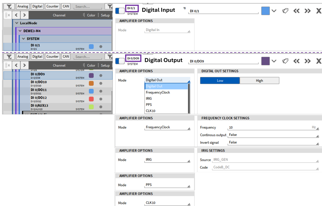
Abb. 7.181: Digital Output Modi für den Chassis-Controller.
