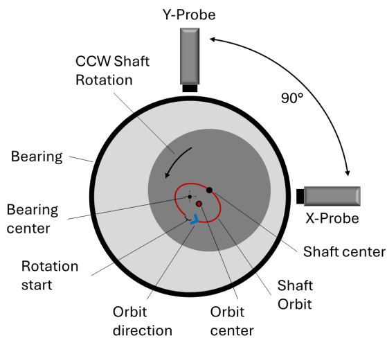
Abb. 8.123: X&Y Probe Anordnung und Orbit-Übersichtsbild
