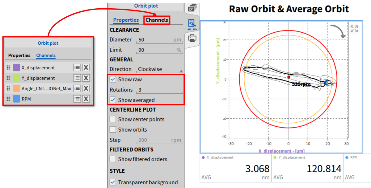
Abb. 8.125: Raw Orbit und Average Orbit
