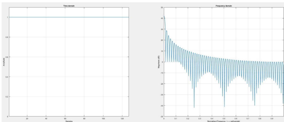
Abb. 8.59: Rechteckfenster in Zeit- und Frequenzbereich (N = 128)
