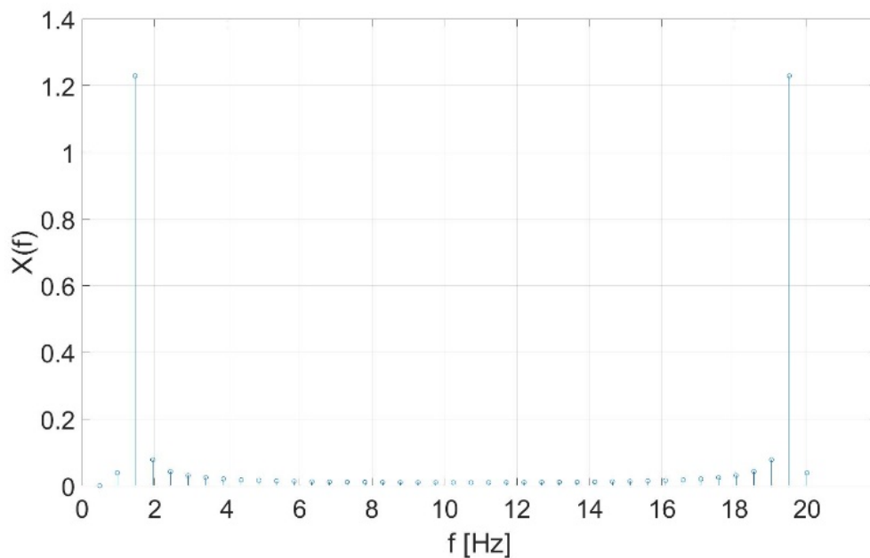
Abb. 8.79: Signal 1 im Frequenzbereich, kein Zero-Padding
