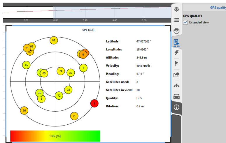
Abb. 8.109: GPS-Qualitäts-Instrument – Erweiterte Sicht ausgewählt
