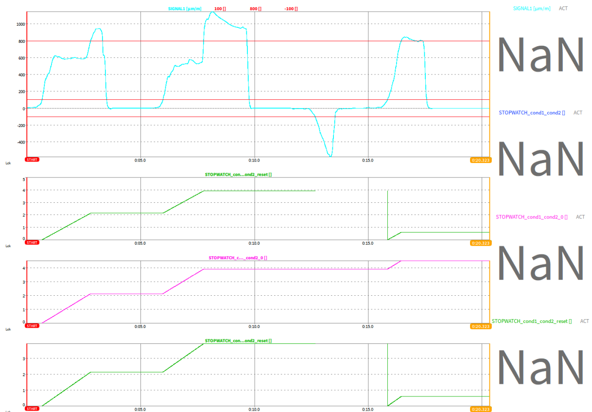
Abb. 7.66: STOPWATCH-Funktion mit Start- und Stop-Bedingung mit definiertem Reset
