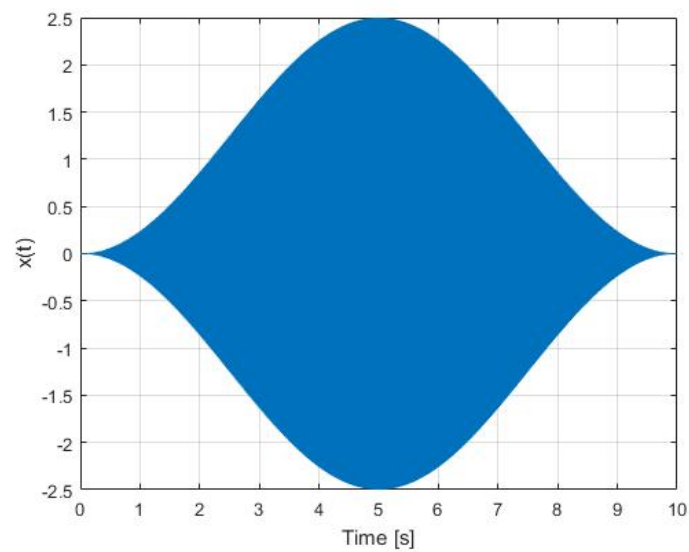
Abb. 8.90: x(t)_{\text{win}} im Zeitbereich; multipliziert mit einem Hanning-Fenster
