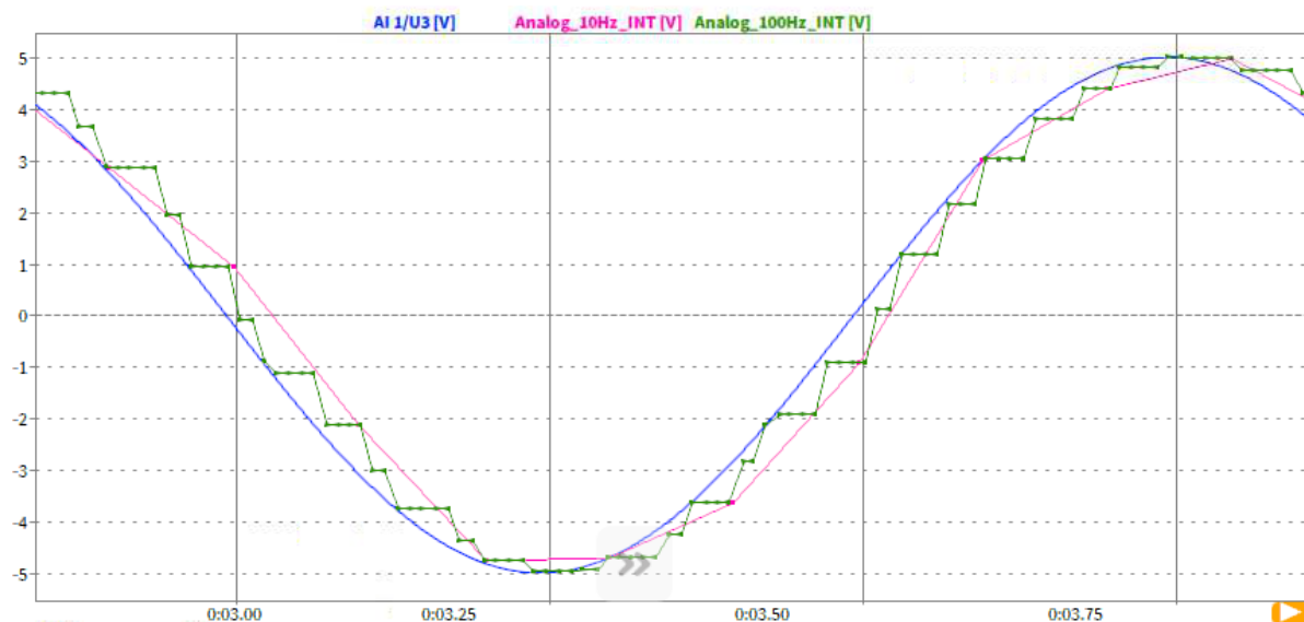
Abb. 7.218: Blau: Analogeingang; Grün: CAN-Ausgang mit einer Verzögerung von 10 ms
