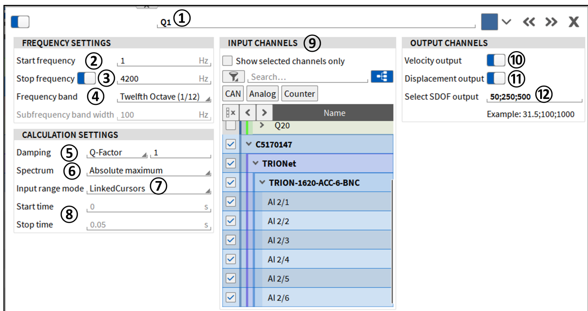
Abb. 7.152: Einstellungen des Shock Response Spectrum-Plugins
