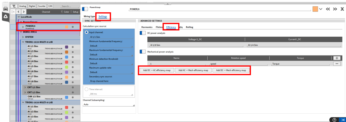
Abb. 7.156: Erstellung eines Matrix Sampler Kanals als Efficiency Map einer zugehörigen Power-Gruppe
