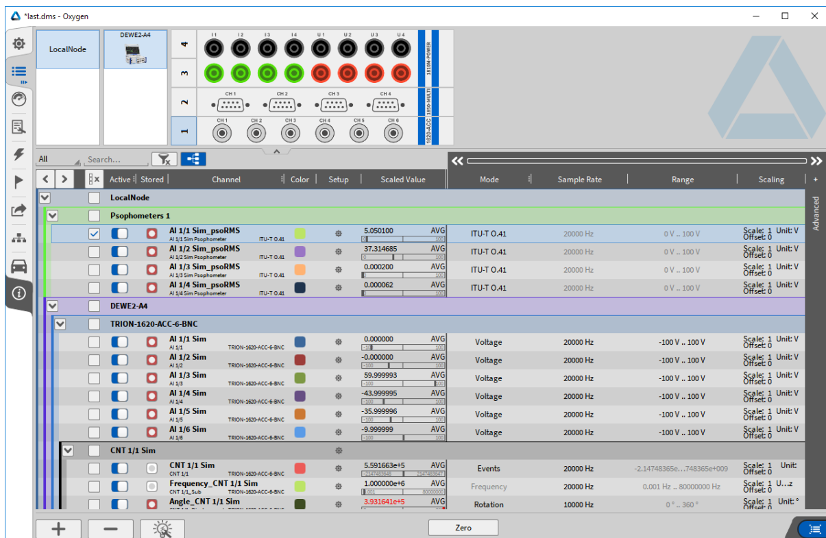
Abb. 7.140: Kanalliste mit der neu erstellten Psophometer-Berechnungsgruppe
