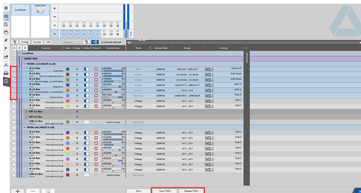
Abb. 7.221: Kanallistenmenü und TEDS-Scan
