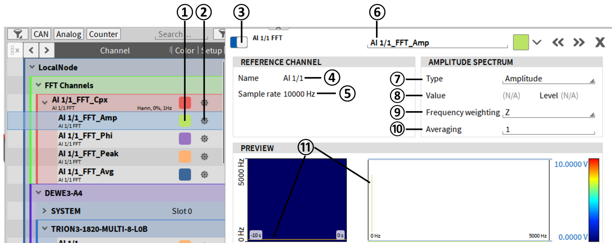
Abb. 7.91: Kanaleinstellungen des Amplitudenspektrums – Übersicht
