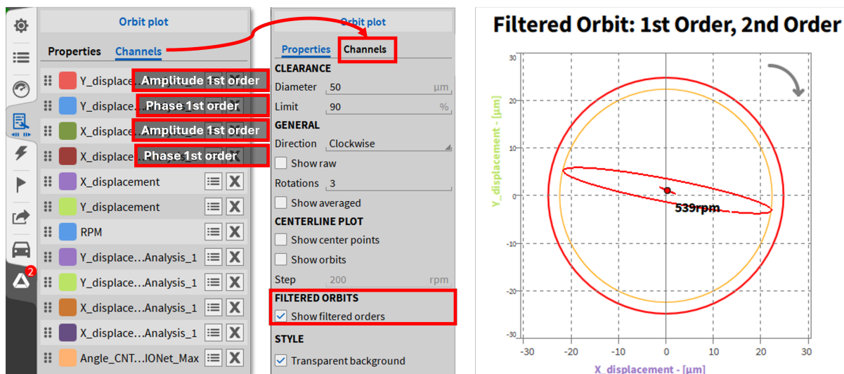
Abb. 8.127: Filtered Orbit Beispiel 1. Und 2. Ordnung aus Ordnungsanalyse
