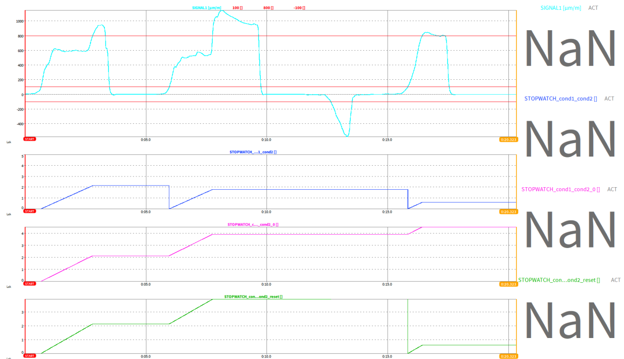
Abb. 7.64: STOPWATCH-Funktion mit Start- und Stop-Bedingung
