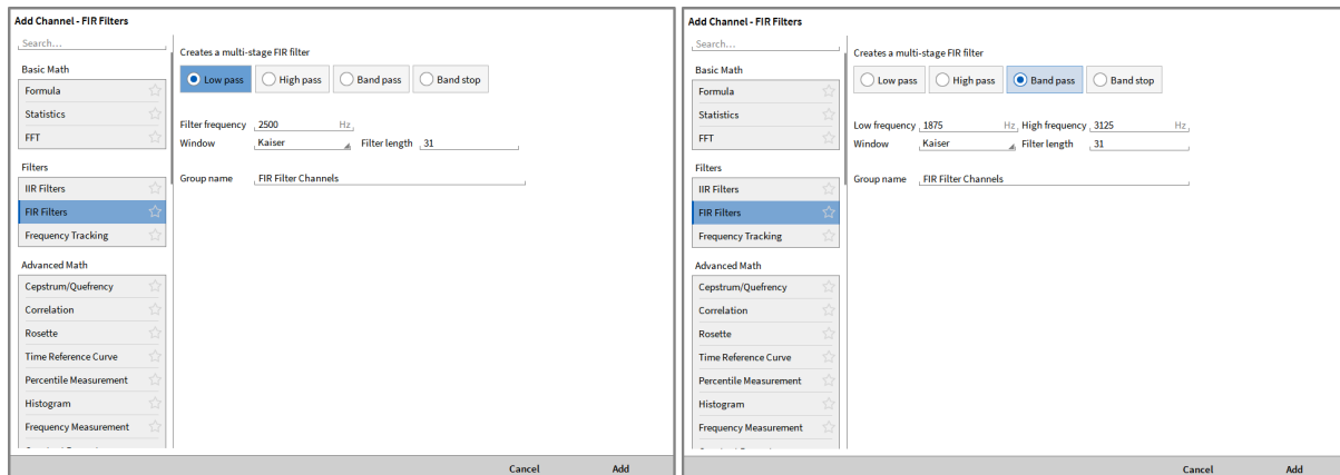
Abb. 7.96: Popup-Fenster zum Erstellen von FIR-Filterkanälen; links: Tiefpass, rechts: Bandpass
