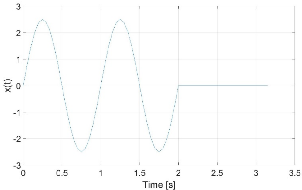
Abb. 8.80: Signal 1 im Zeitbereich, Zero-Padding auf 64 Samples
