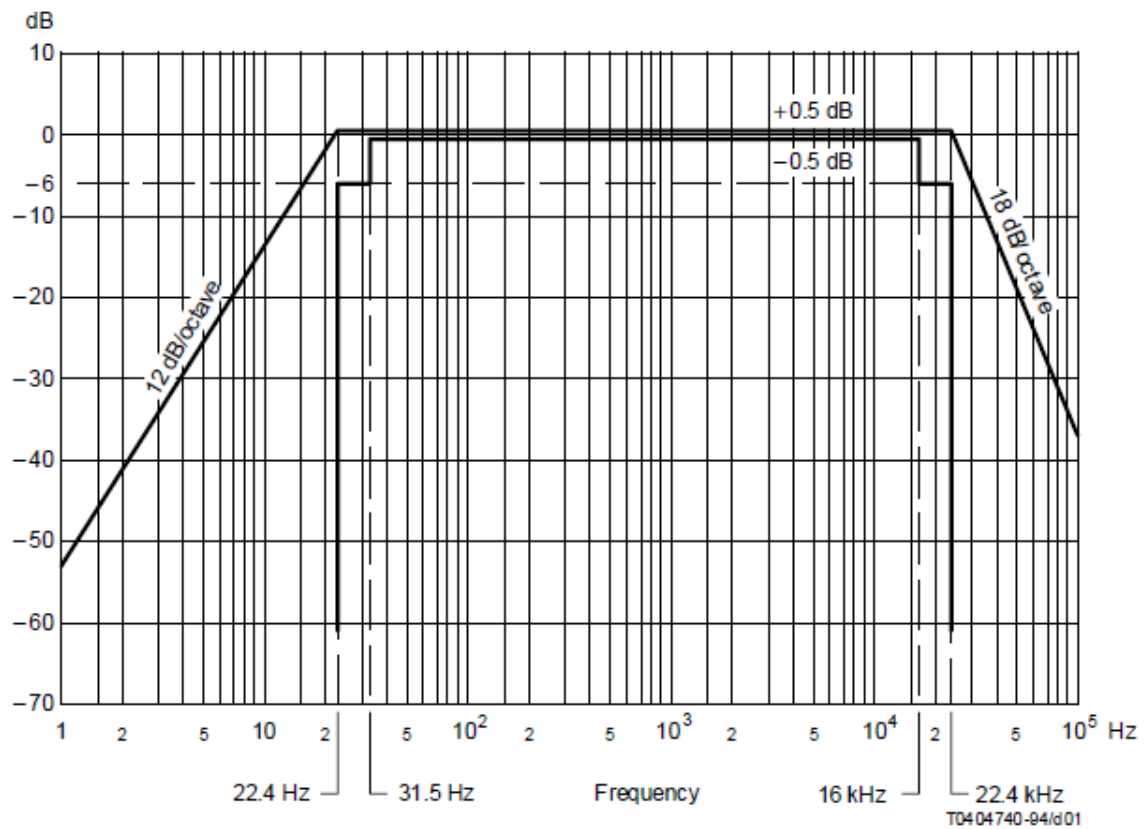
Abb. 7.146: Charakteristika der Frequenzantwort für ungewichtete Messungen
