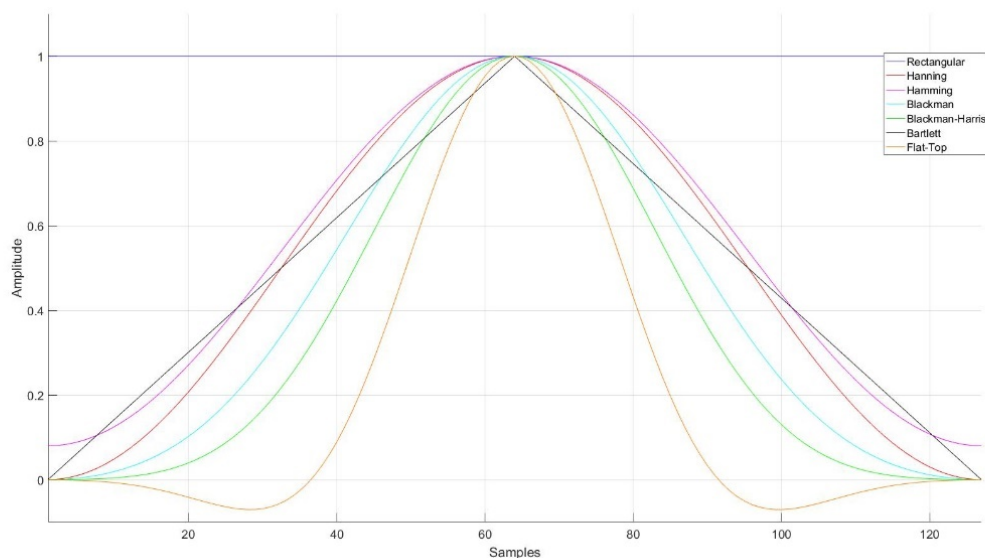
Abb. 8.61: Vergleich der verschiedenen Fensterfunktionen im Zeitbereich (N = 128)
