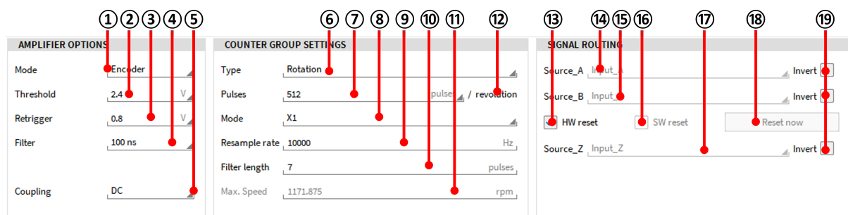
Abb. 7.196: Kanaleinstellungen für einen TRION-CNT Kanal im Encoder-Modus
