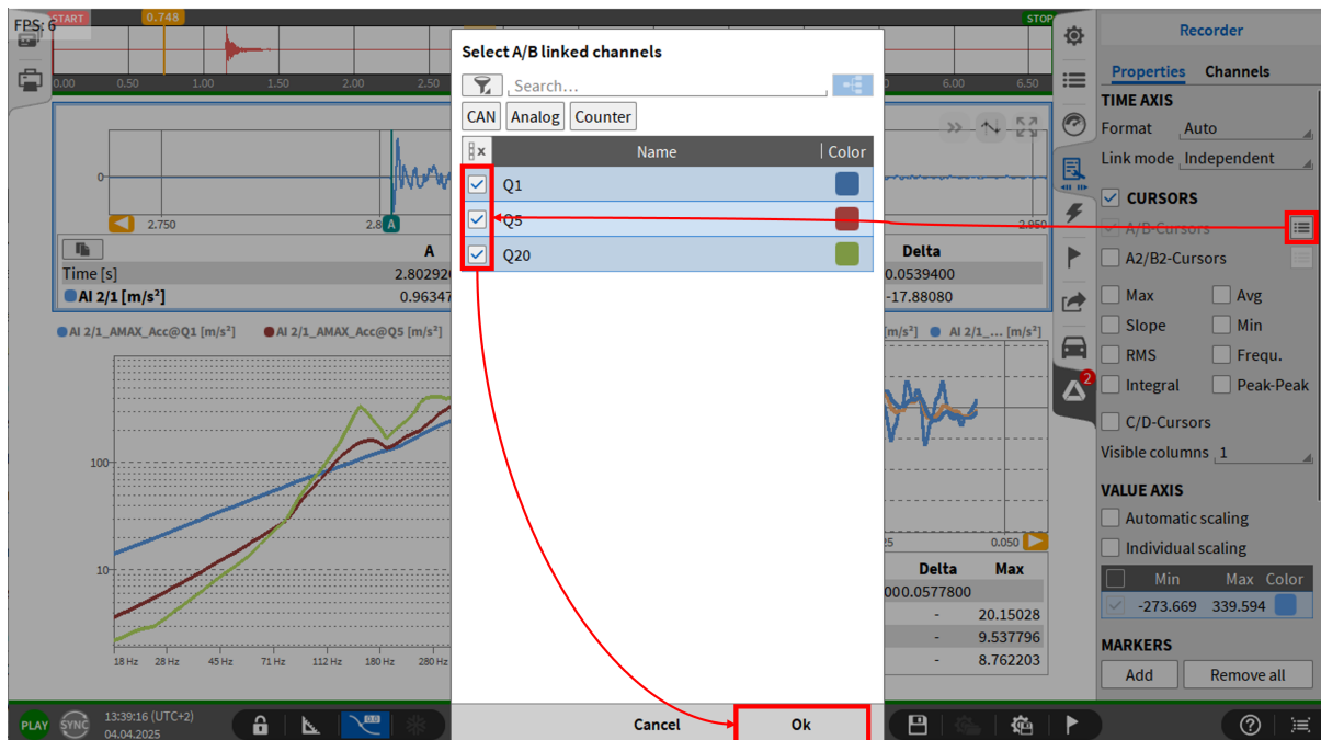
Abb. 7.153: Verlinken des AB-Zeiger als Zeitbereich für die SRS-Kalkulation
