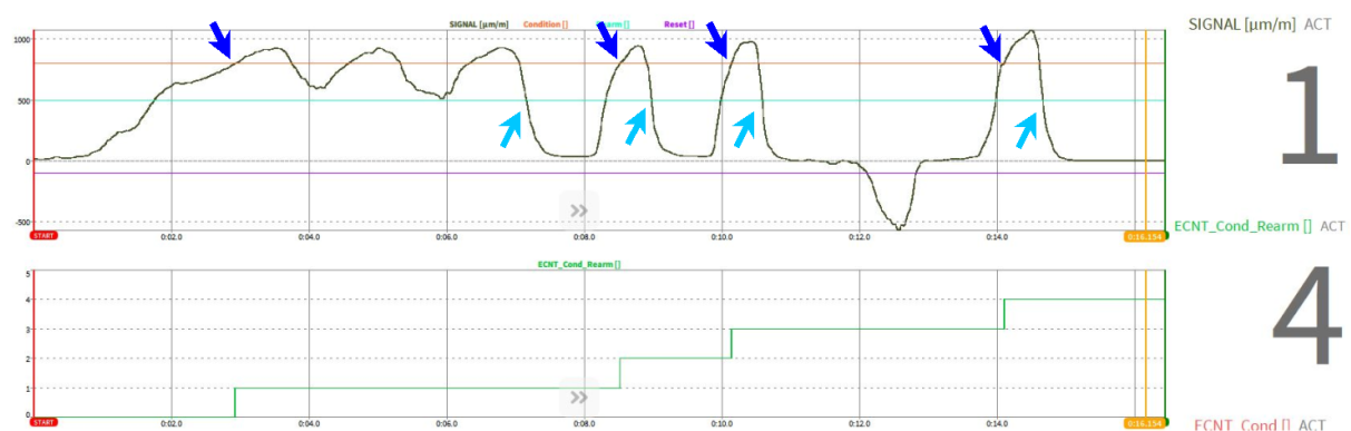
Abb. 7.58: ECNT-Funktion mit Bedingung und Rearm
