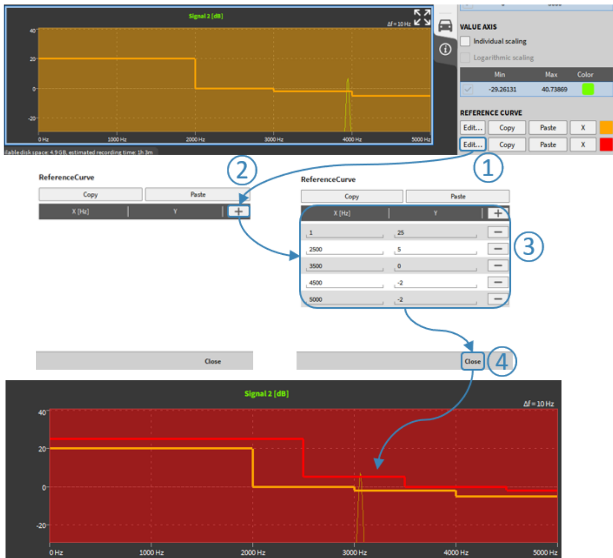
Abb. 8.69: Erstellung einer roten Referenzkurve
