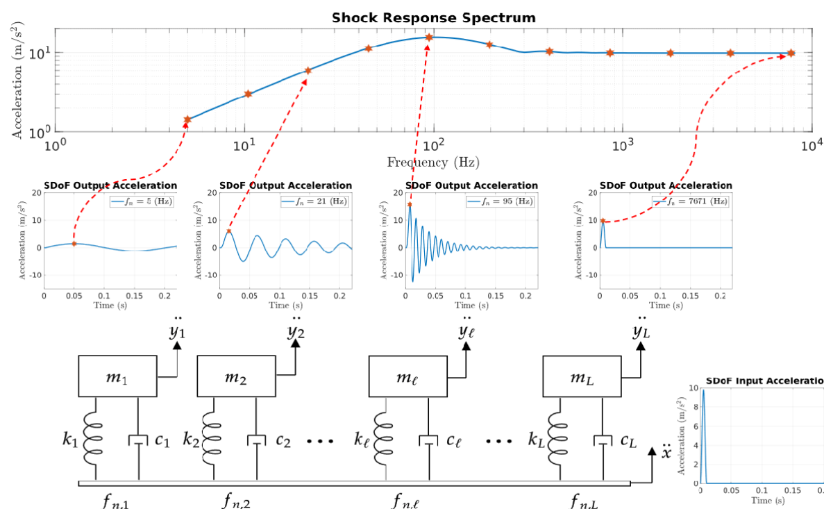
Abb. 7.150: Schematisches Verfahren zur Berechnung eines Schockantwortspektrums
