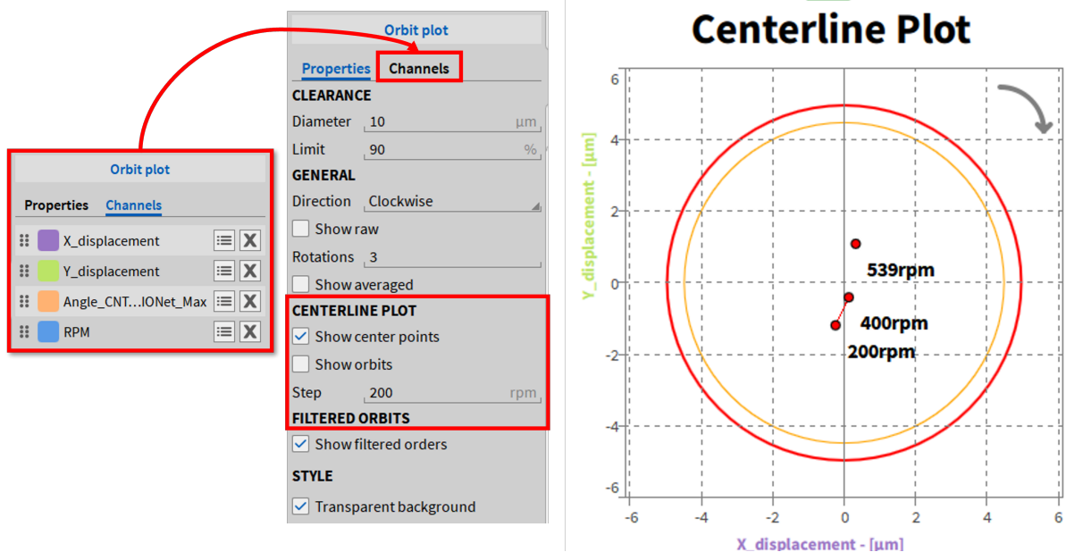
Abb. 8.126: Centerline Plot Beispiel
