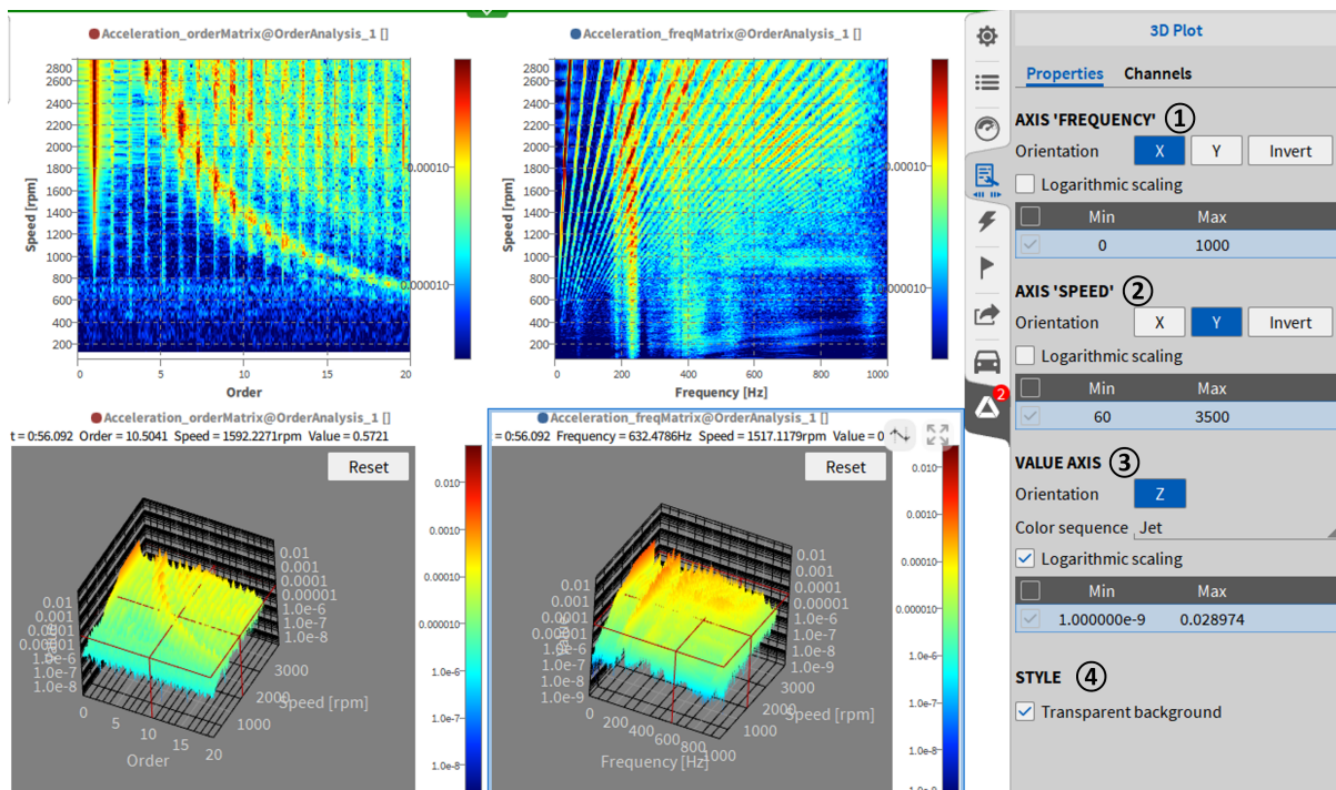
Abb. 8.44: 3D-Plot Beispiel und Instrumente Eigenschaften
