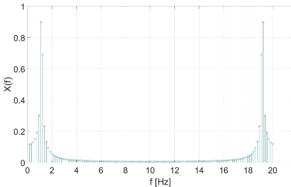
Abb. 8.85: Signal 2 im Frequenzbereich, kein Zero-Padding
