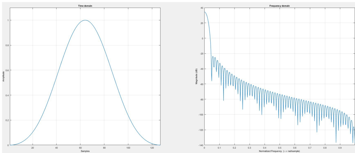
Abb. 8.60: Blackman-Fenster in Zeit- und Frequenzbereich (N = 128)
