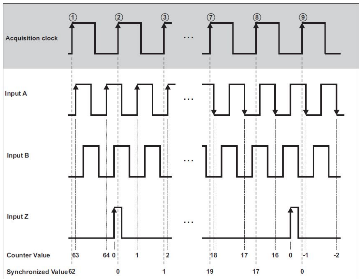
Abb. 7.190: Quadratur-Encoder mit Kanal Z
