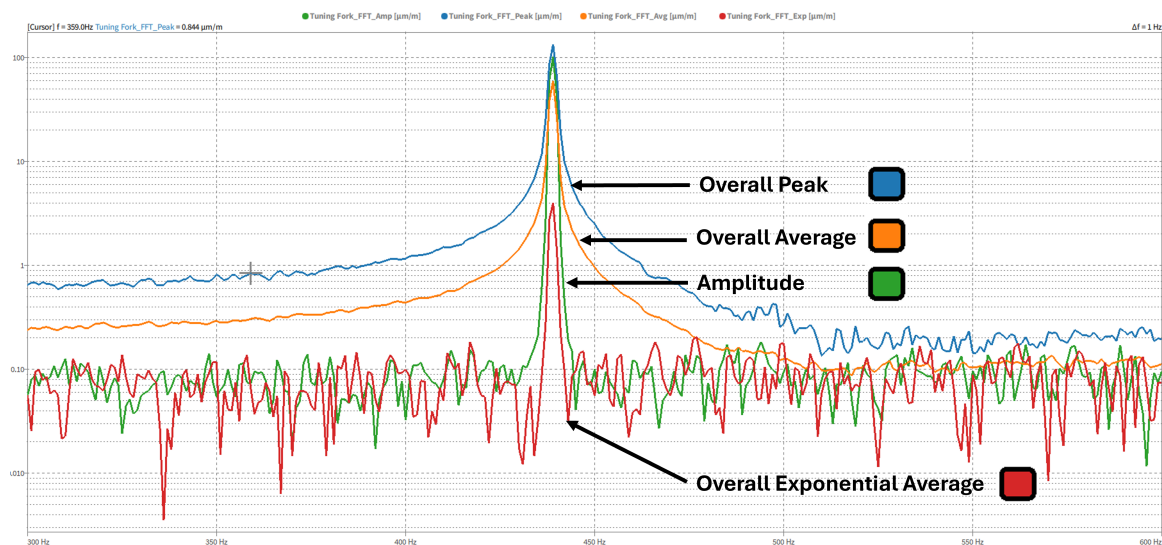
Abb. 7.93: Beispiel für Amplituden, Gesamtspitzenwert, Gesamtmittelwert und exponentiellen Mittelwert in der Spektralansicht
