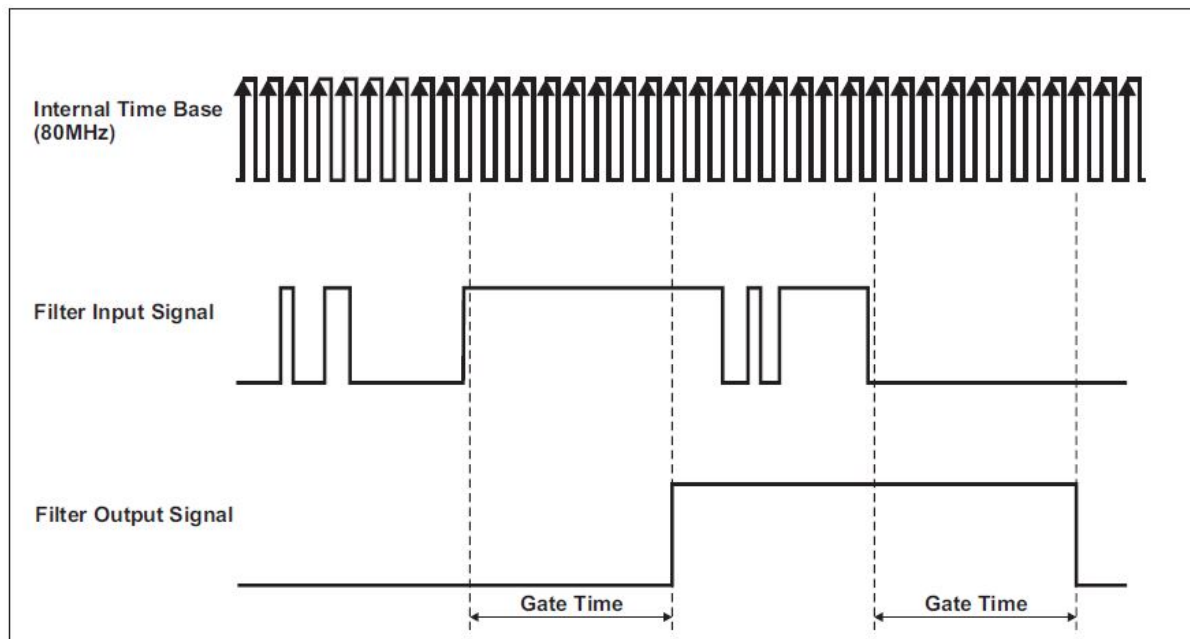
Abb. 7.198: Eingangssignal mit Chatter
