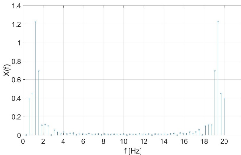
Abb. 8.81: Signal 1 im Frequenzbereich, Zero-Padding auf 64 Samples
