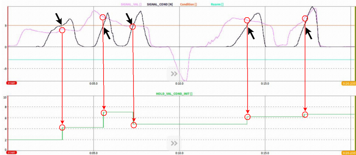
Abb. 7.61: HOLD-Funktion mit Bedingung und initialem Wert
