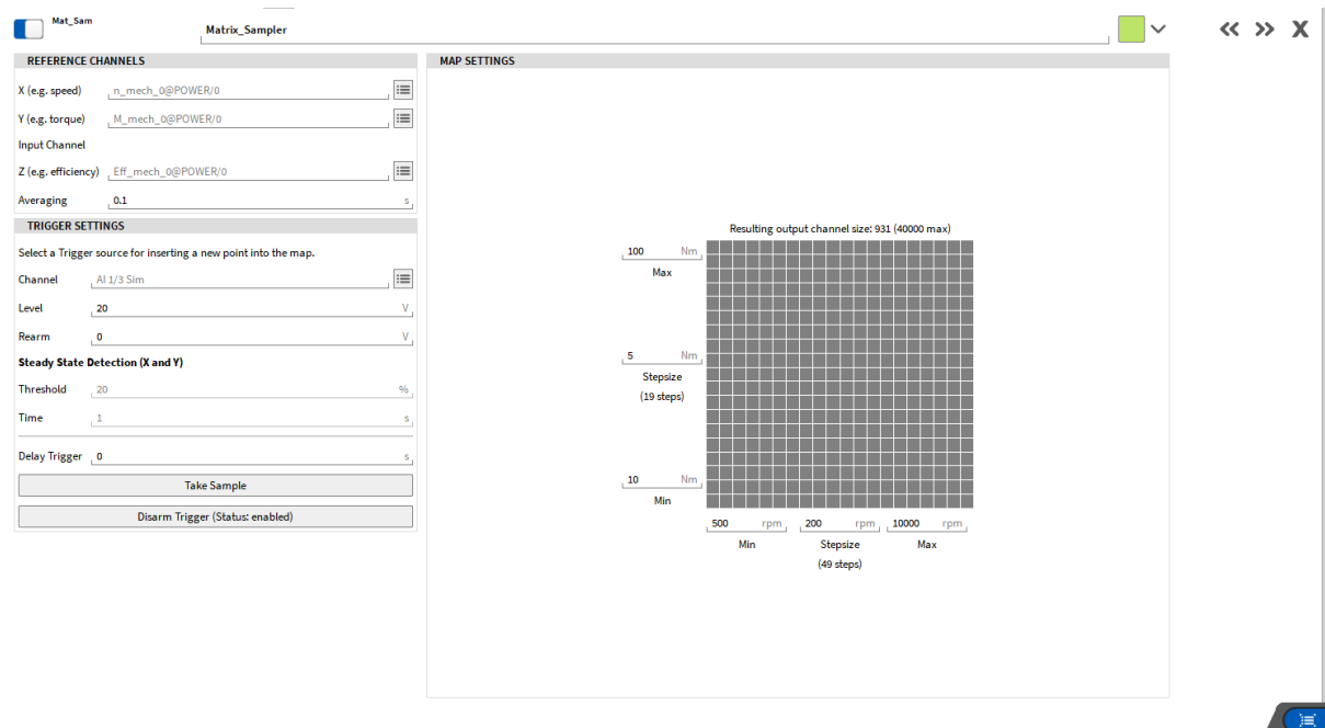
Abb. 7.158: Kanaleinstellungen eines Matrix Sampler Kanals
