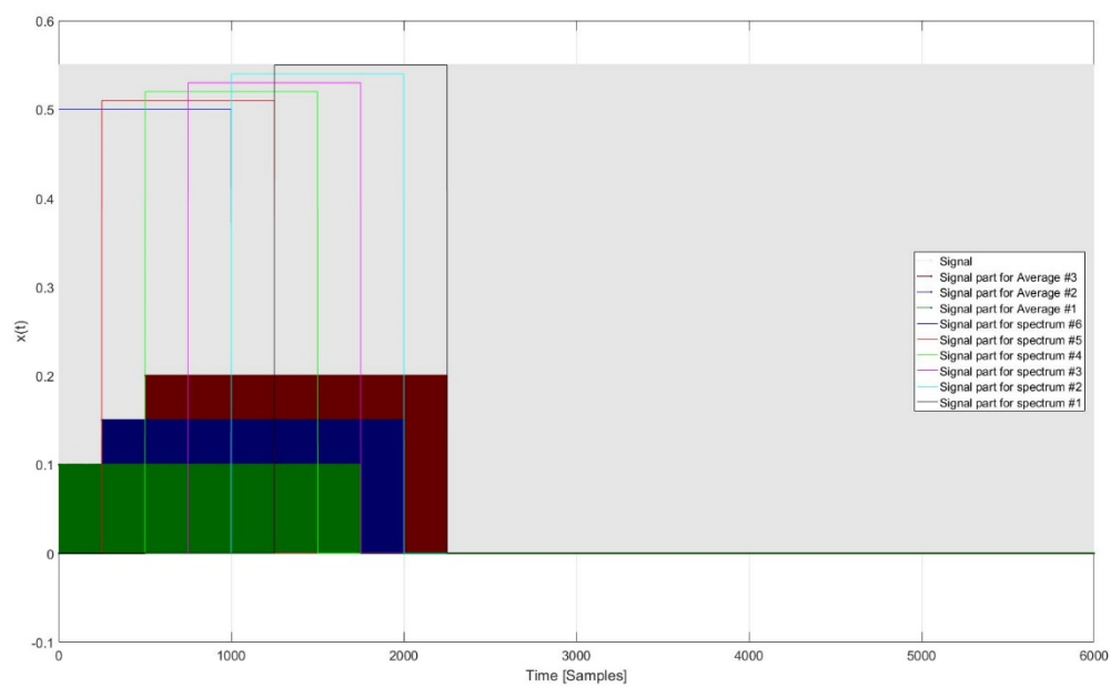
Abb. 8.97: Zerlegung des Signals im Zeitbereich für die Mittelung von 4 Spektren und 75 % Überlappung
