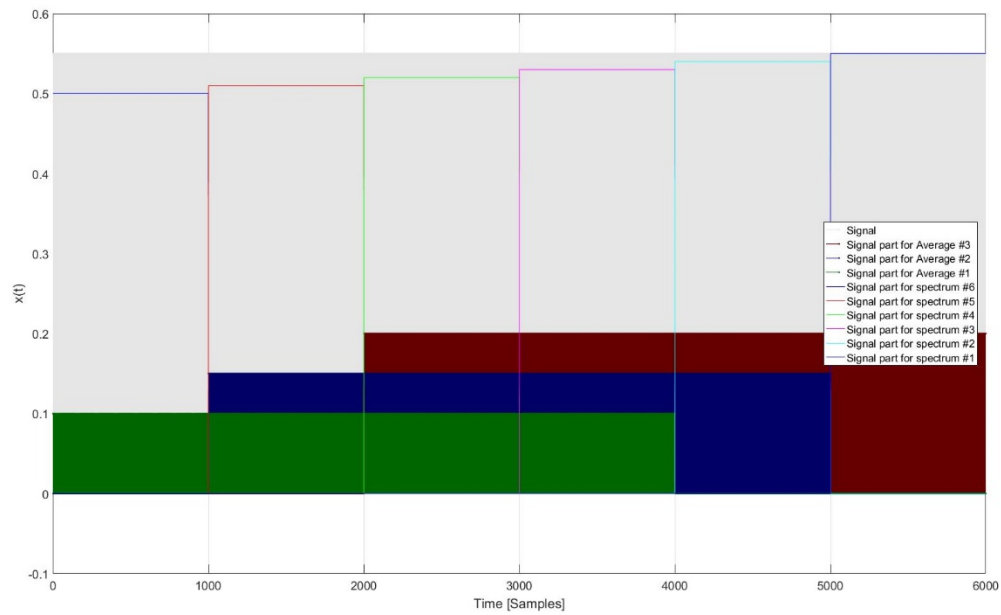
Abb. 8.96: Zerlegung des Signals im Zeitbereich für die Mittelung von 4 Spektren und 0 % Überlappung
