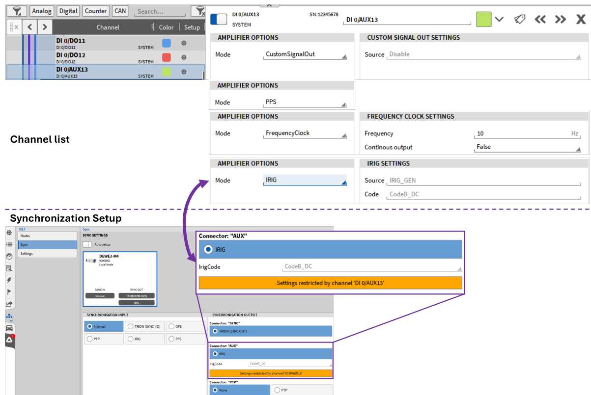
Abb. 7.182: AUX Ausgangs Modi für den Chassis-Controller.
