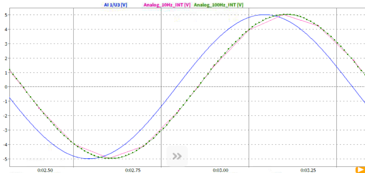
Abb. 7.217: Blau: Analogeingang; Grün: CAN-Ausgang mit einer Verzögerung von 70 ms (Standardwert)
