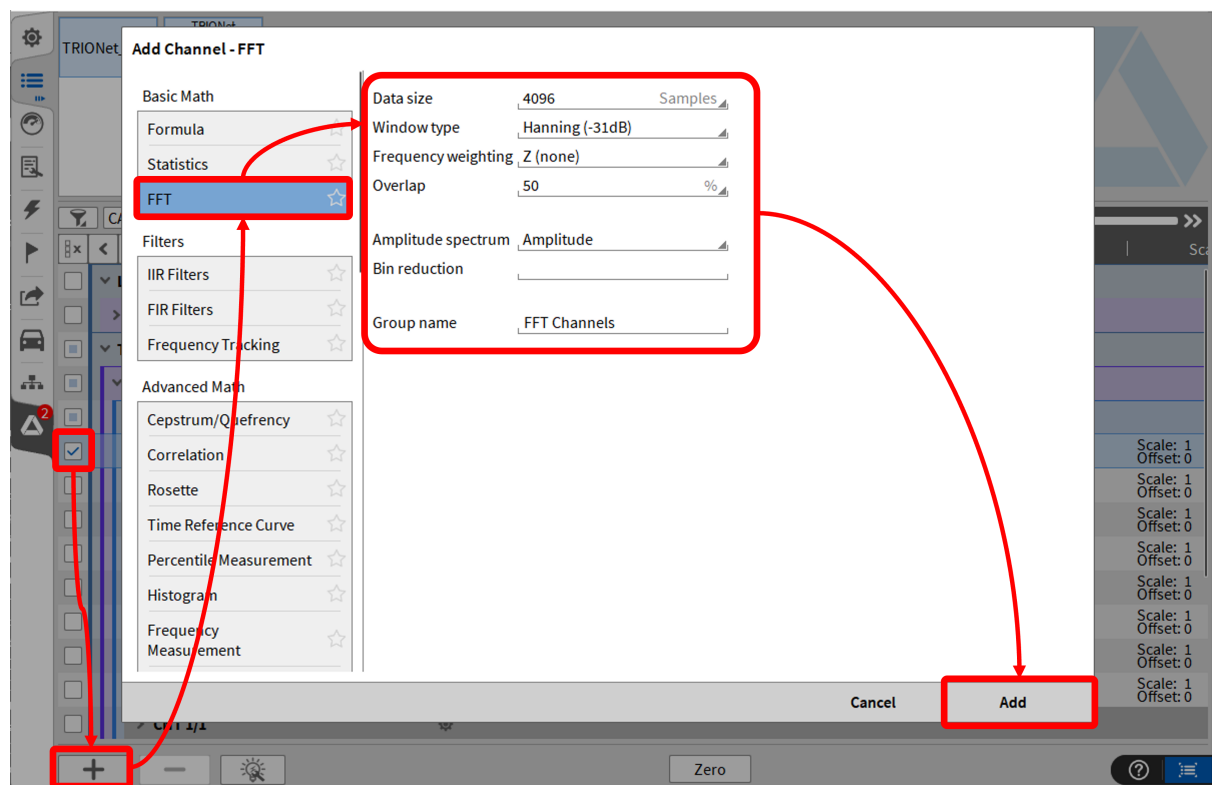
Abb. 7.88: Pop-up-Fenster zur Erstellung eines FFT-Kanals
