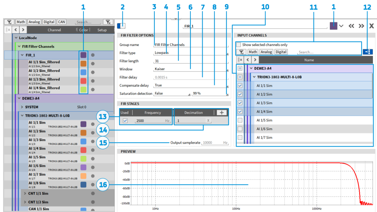
Abb. 7.97: FIR - FIR Einstellungen
