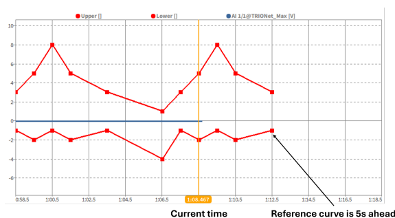
Abb. 7.120: Beispiel obere und untere Zeitreferenzkurve mit 5 s Vorauszeit (Zeit Offset)
